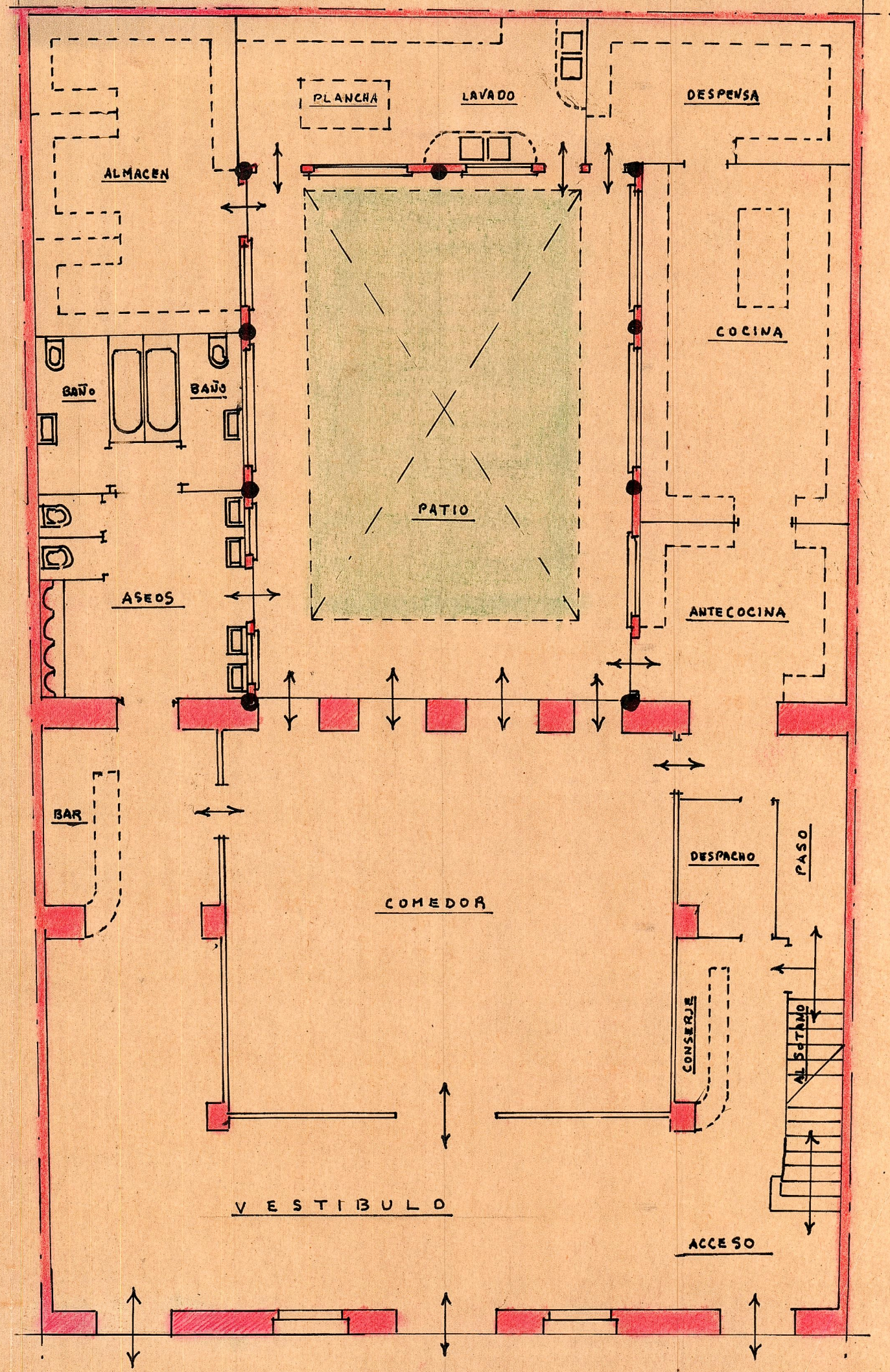
PLANTA BAJA
