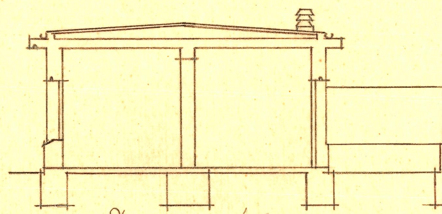
Sección por A-B
