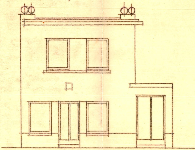
Fachada
