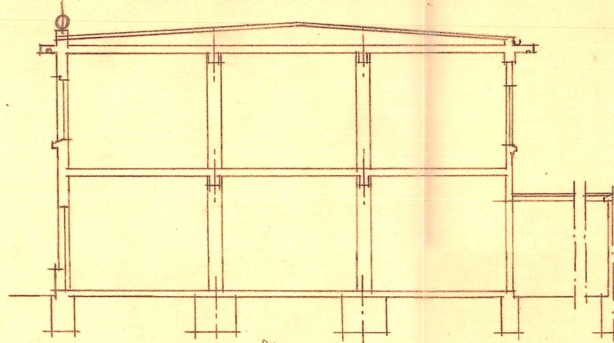
Sección
