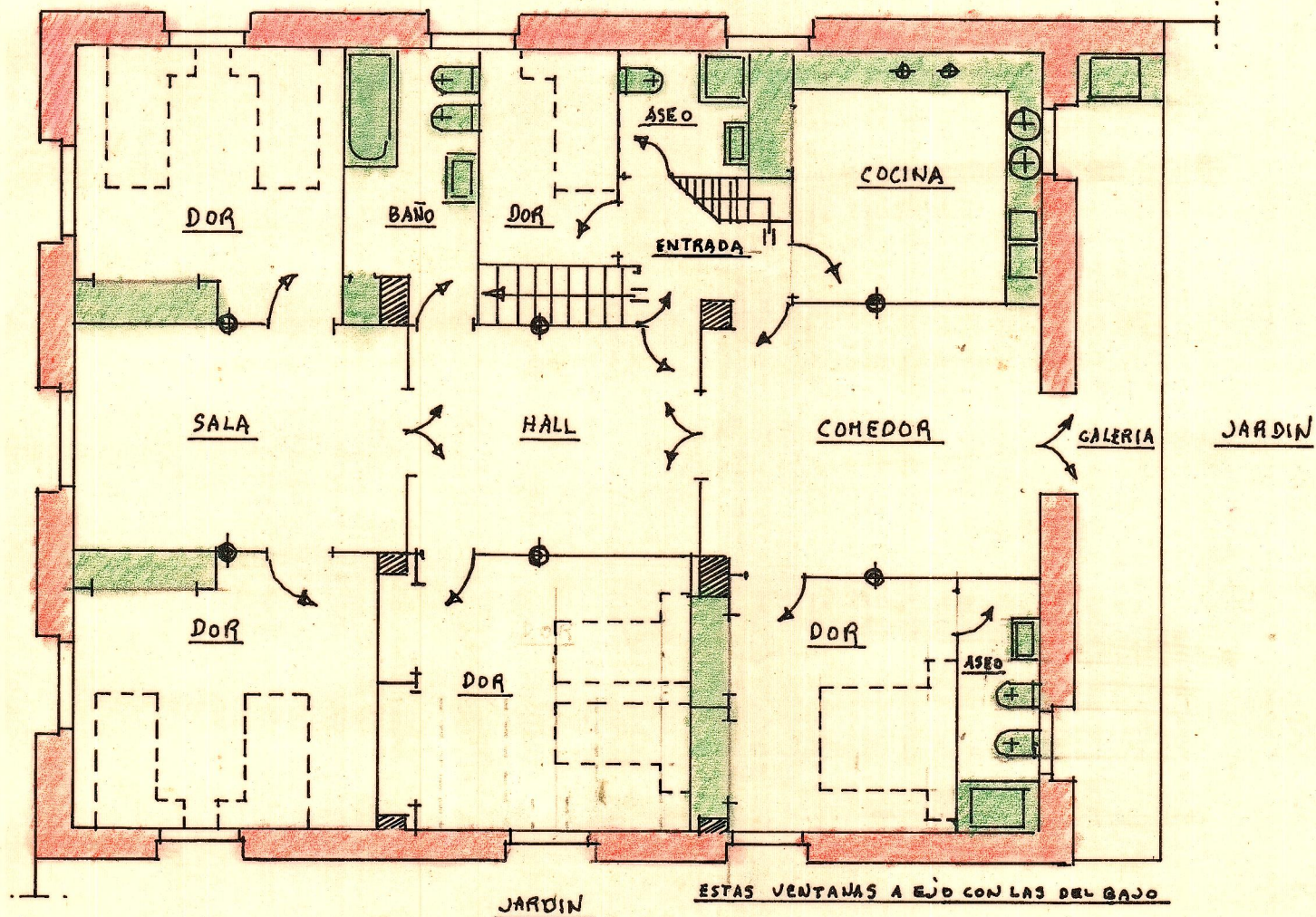
PLANTA ALTA - E - 11100
