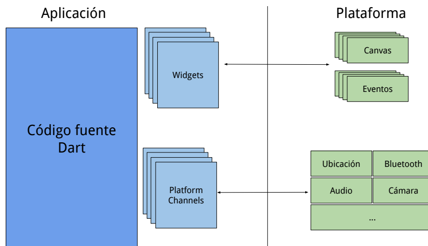
Figura 4.1: Diagrama de renderización de Flutter [17]
