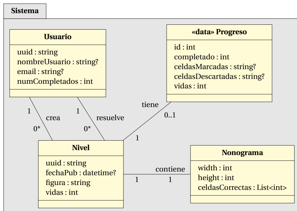
Figura 3.1: Diagrama del modelo de dominio
