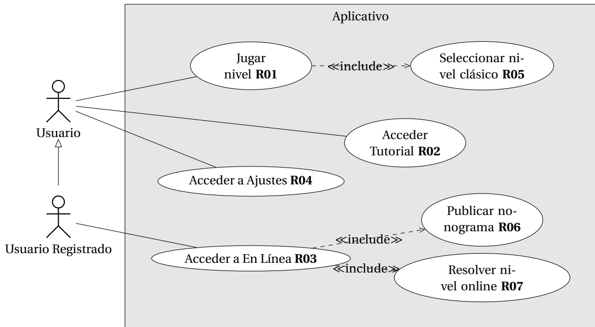
Figura 3.3: Diagrama de casos de usos principales
