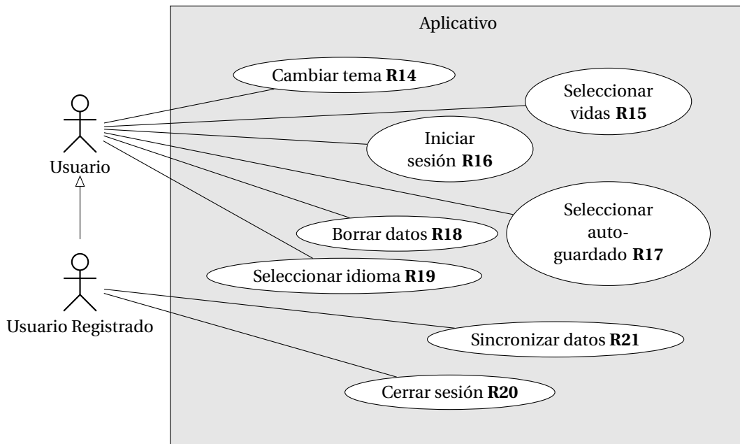
Figura 3.5: Diagrama de casos de ajustes
