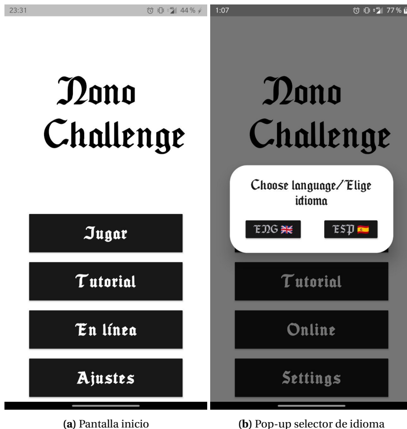
Figura 8.1: Pantallas iniciales
