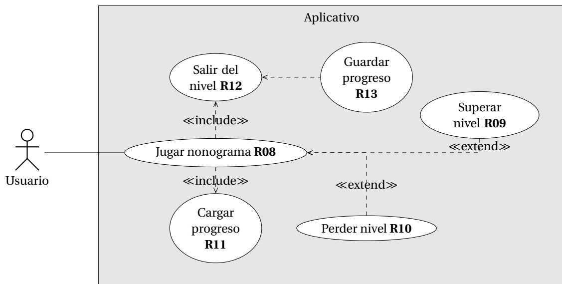
Figura 3.4: Diagrama de casos de usos en pantalla de resolución de nivel
