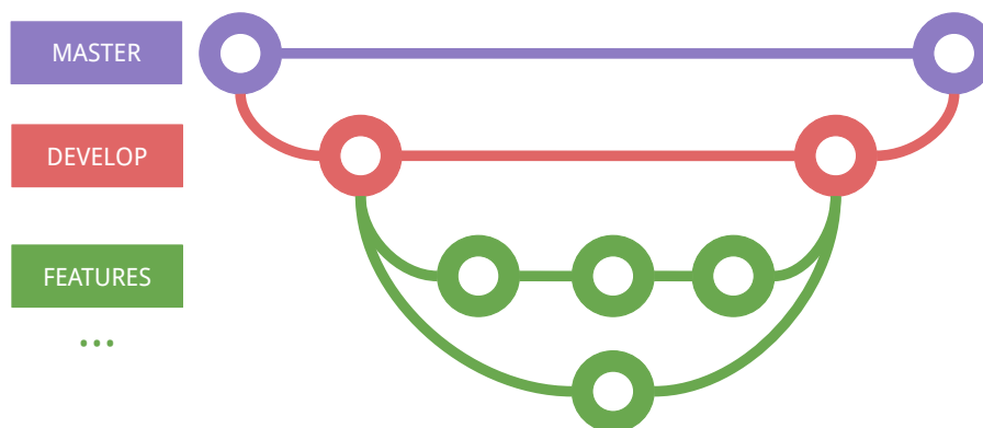
Figura 4.4: Diagrama del funcionamiento de GitFlow
