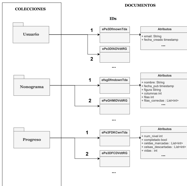
Figura 4.3: Diagrama de estructura de datos de Firestore
