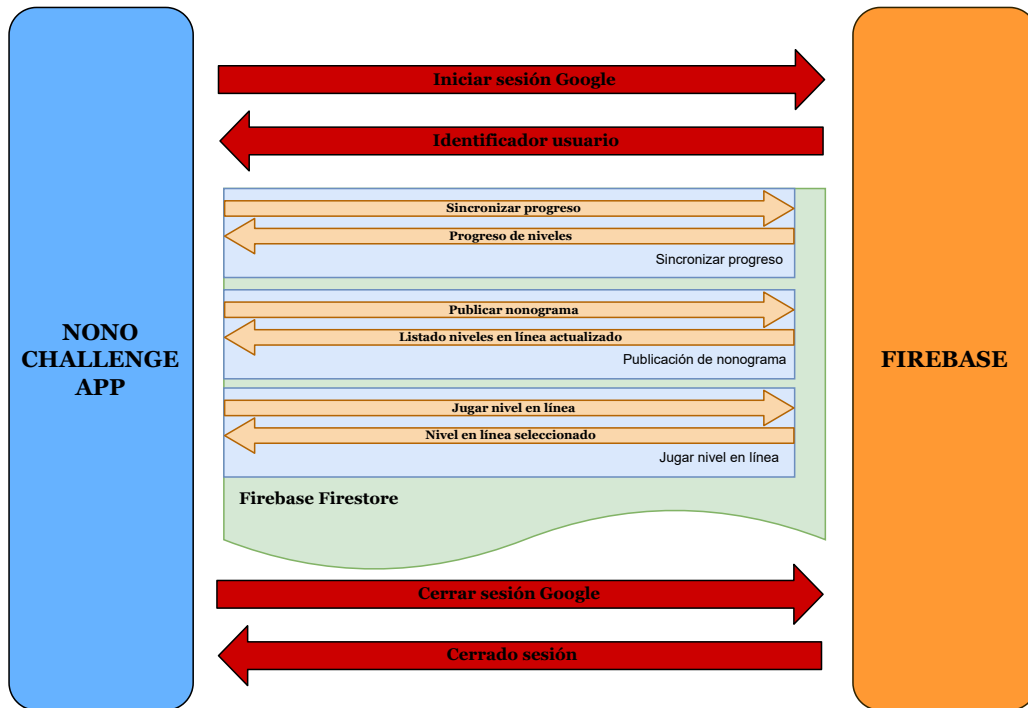
Figura 4.2: Diagrama de flujo con Firebase
