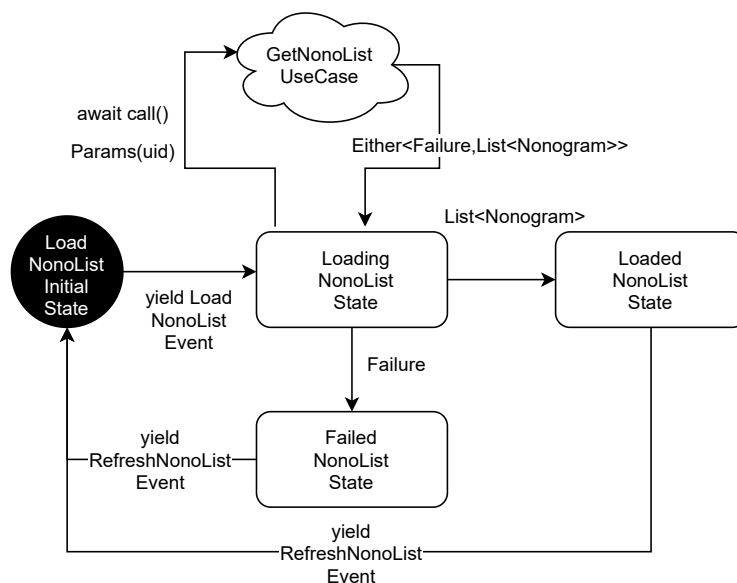
Figura 5.7: Diagrama de estado de la funcionalidad Lista de nonogramas en línea
