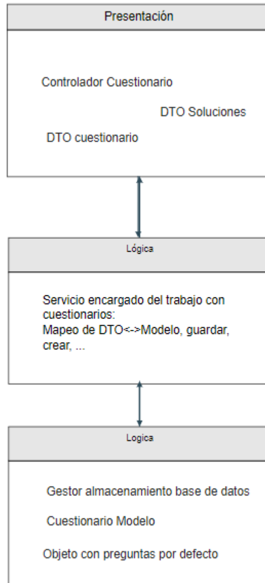
Figura 18 Estructura del cuestionario (primera versión)
