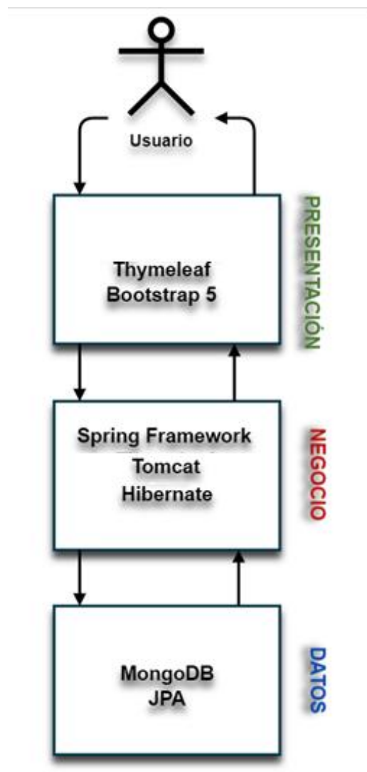
Figura 3 Arquitectura detallada de la aplicación
