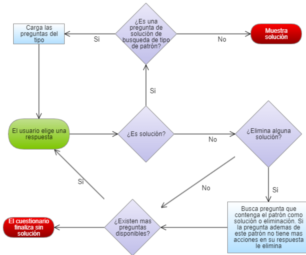
Figura 24 Flujo del algoritmo de sugerencia de patrón
