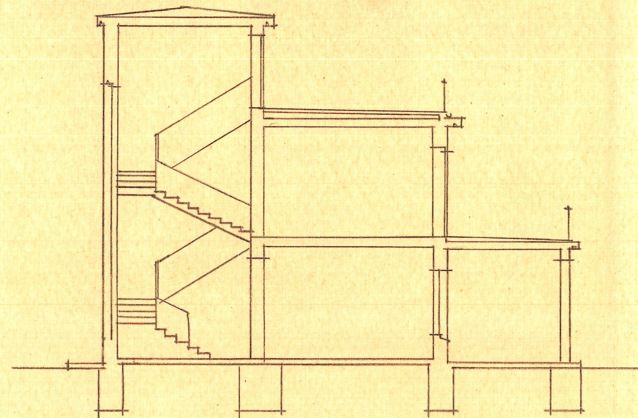
Sección transversal
