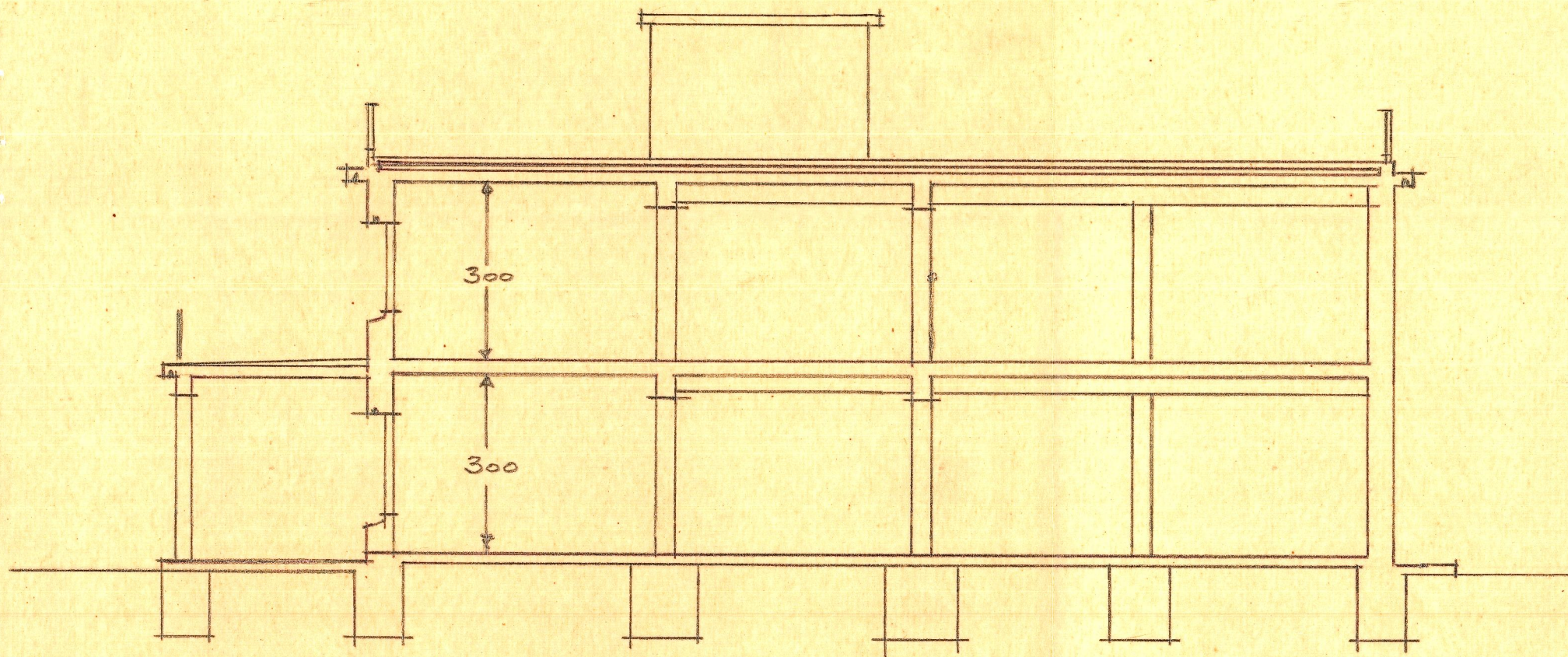
Sección longitudinal
