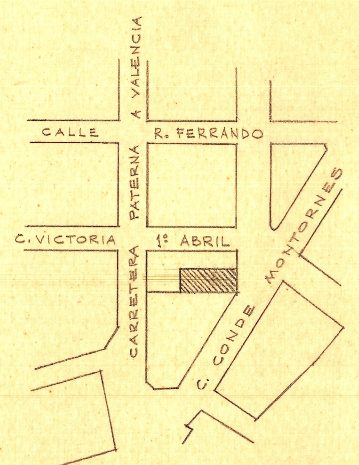
Implantación E=1:2000
