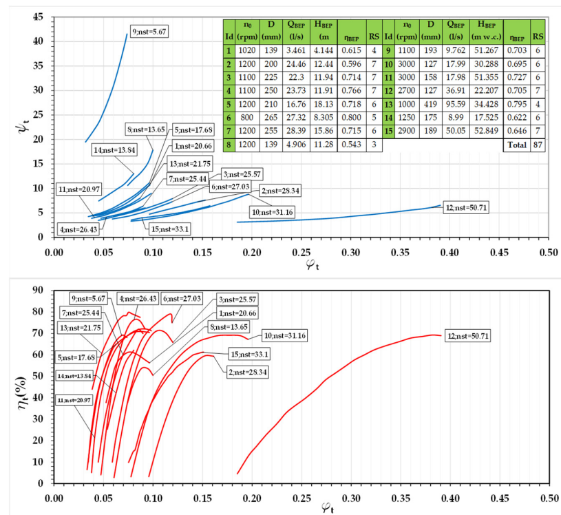
Figure 3. Experimental database. ID1 [23]; ID2-ID4 [24]; ID5-ID7 [21]; ID8 [25]; ID9 [26]; ID10-ID12 [27]; ID13 [28]; ID14 [2]; ID15 [3].
