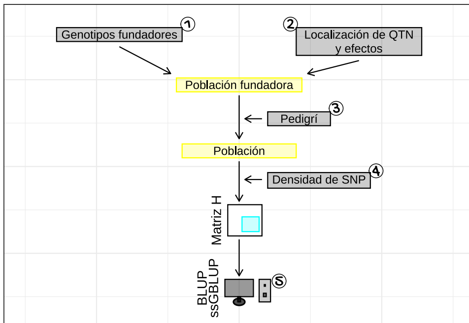
Figura 4.5: Esquema de predicción usando simulación con el paquete SeqBreed . Figura adaptada de Pérez-Enciso, Ramírez-Ayala, y Zingaretti (2020).
