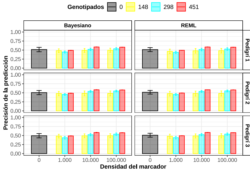
Figura 5.5: Precisión de la predicción con tamaños crecientes en el número de marcadores y de individuos genotipados en la simulación ancestral para los tres pedigrís simulados. Las barras representan la media de la precisión de la predicción de las 10 réplicas de cada pedigrí y las barras de error representan el desvío estándar como medida de variabilidad.
