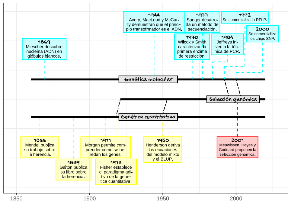
Figura 2.1: Cronología de las disciplinas de la genética molecular y la genética cuantitativa. Varios descubrimientos permitieron la conexión entre ambas disciplinas lo que permitió el desarrollo de la selección genómica. Figura adaptada de Nelson, Pettersson, y Carlborg (2012).
