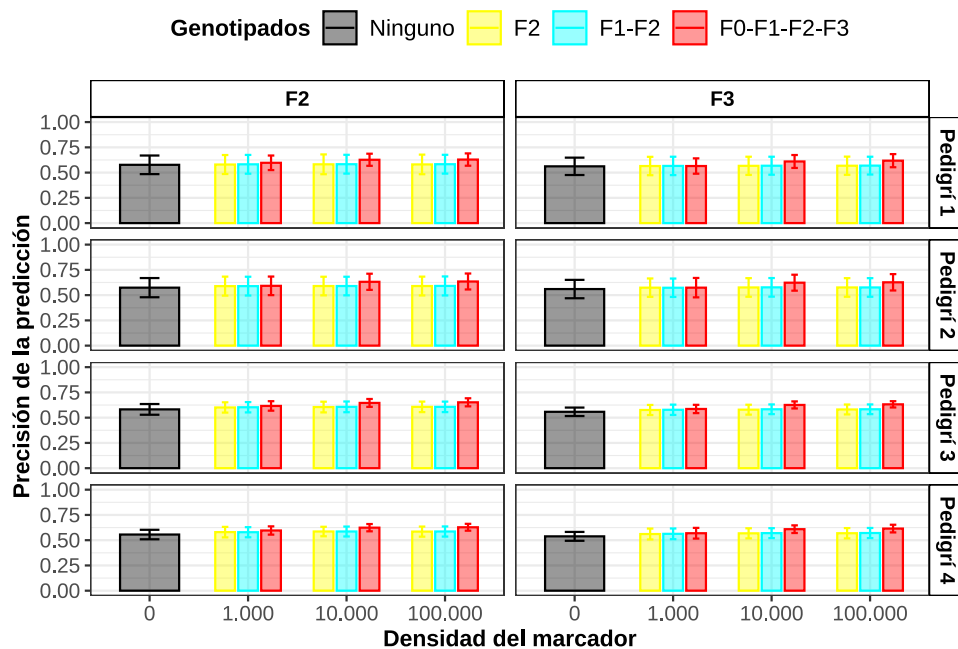
Figura 5.6: Precisión de la predicción con tamaños crecientes en el número de marcadores y de individuos genotipados en la simulación de descendientes para los cuatro pedigrís simulados. Las barras representan la media de la precisión de la predicción de las 10 réplicas de cada pedigrí y las barras de error representan el desvío estándar como medida de variabilidad.
