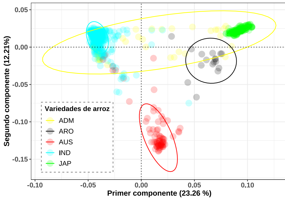
Figura 4.1: Análisis de componentes principales en datos de arroz. Los puntos y las circunferencias de color representan los distintos grupos varietales disponibles: tipo intermedio o mezclado (ADM), aromático (ARO), aus (AUS), indica (IND) y japónica (JAP).
