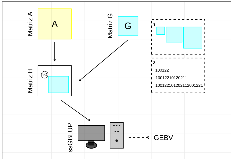
Figura 4.4: Esquema de construcción de la matriz H a partir de la matriz A y la matriz G , con base en diferentes subconjuntos de datos (o matrices G ). El recuadro 1 representa tres matrices G con distinta dimensión dado el número de individuos genotipados y el recuadro 2 representa tres diferentes densidades de SNP, para cada uno de las tres matrices del recuadro 1.
