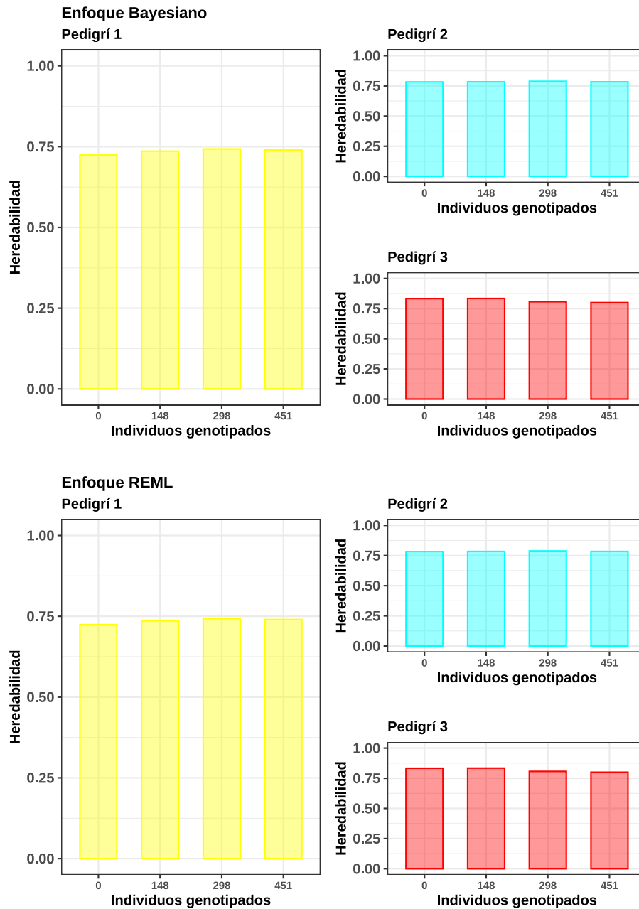
Figura 5.4: Estimaciones de componentes de varianza y de heredabilidad mediante enfoques Bayesiano y REML, para el carácter tiempo de floración con tamaños crecientes en el número de individuos genotipados con una densidad aproximada de 100.000 marcadores. Las barras representan la media del valor de heredabilidad obtenida de las 10 réplicas de cada pedigrí y Pedigrí 1-2-3 son los tres pedigríes simulados mediante simulación ancestral.
