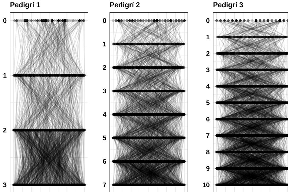
Figura 4.3: Ejemplo de pedigrís generados en la primera replica. En cada pedigrí se generaron distintas generaciones por encima de los individuos de la población fundadora. El número de individuos totales en cada pedigrí fueron: 751 individuos en el pedigrí 1, 1.661 en el pedigrí 2 y 2.451 en el pedigrí 3.
