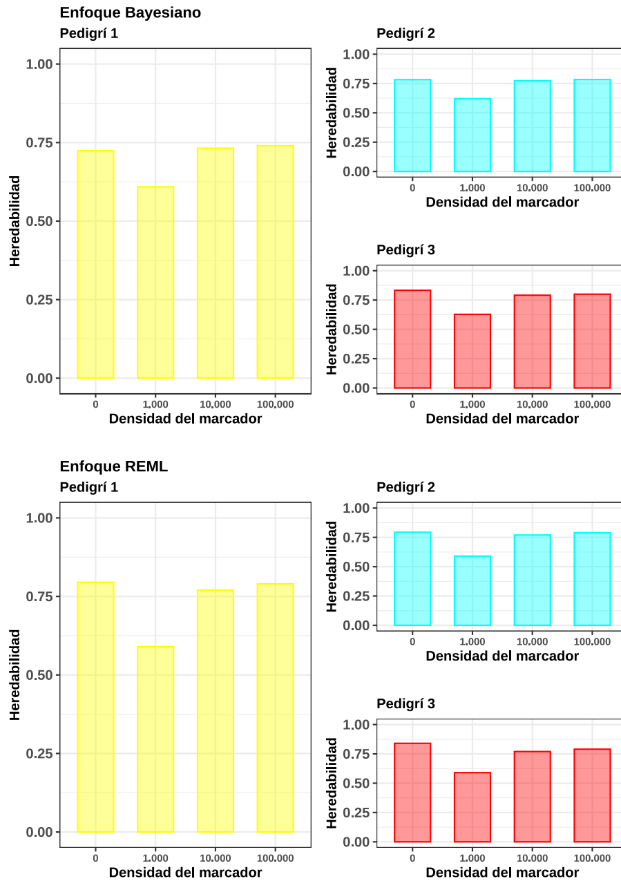
Figura 5.3: Estimaciones de componentes de varianza y de heredabilidad mediante enfoques Bayesiano y REML, para el carácter tiempo de floración con tamaños crecientes en el número de marcadores en 451 individuos genotipados (excepto con una densidad de 0 que correspondería a ningún individuo genotipado). Las barras representan la media del valor de heredabilidad obtenida de las 10 réplicas de cada pedigrí y Pedigrí 1-2-3 son los tres pedigrís simulados mediante simulación ancestral.
