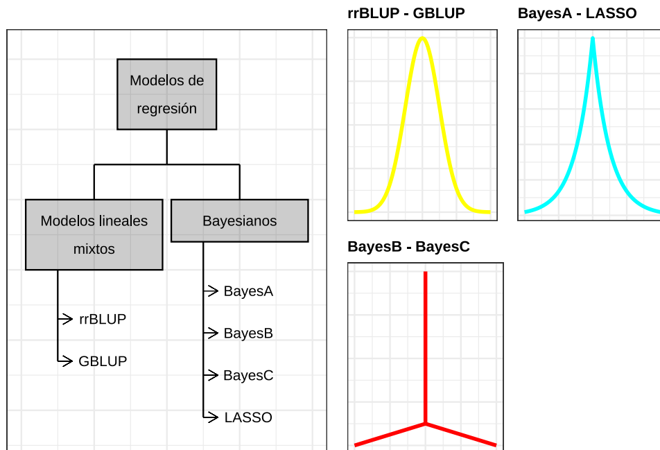
Figura 2.5: Enfoques estadísticos de la selección genómica. Cada uno de estos enfoques suponen distintas distribuciones de efectos de los marcadores sobre el carácter. Figura adaptada de de los Campos et al. (2013) y de Tong y Nikoloski (2021).
