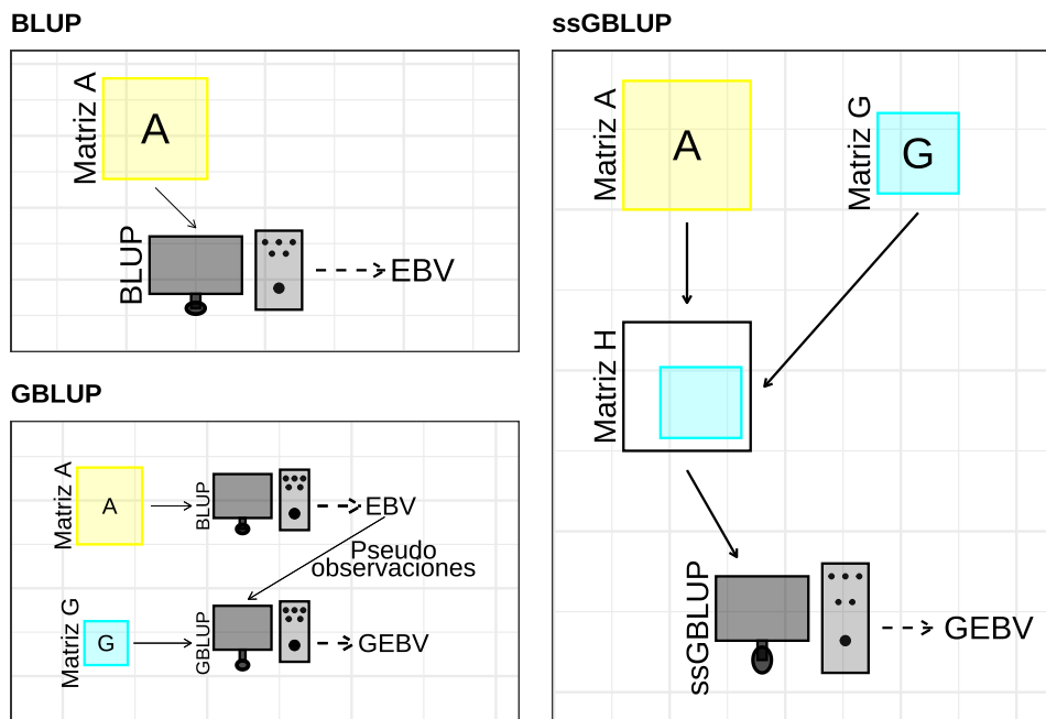
Figura 2.7: Esquema de comparación del BLUP, GBLUP y ssGBLUP. El GBLUP es un proceso de tres pasos en el que los individuos, con base en su información fenotípica y de pedigrí, son evaluados inicialmente mediante el BLUP; luego, a partir de los pseudo-fenotipos resultantes de esta evaluación inicial, se lleva a cabo un análisis genómico de los individuos genotipados mediante el GBLUP. En el ssGBLUP se simplifica este proceso al incorporar la información genómica (la matriz G) desde el primer paso.
