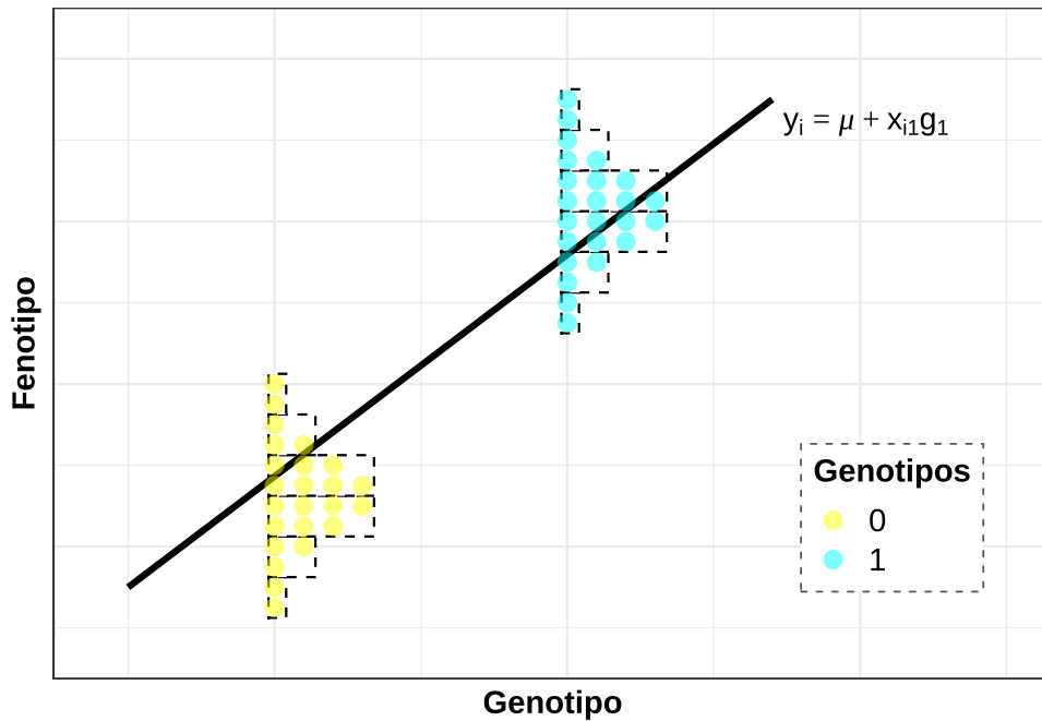
Figura 2.4: Relación genotipo-fenotipo de individuos (círculos amarillo y azul) para un solo marcador. Y_i y x_{i1} denotan los fenotipos y genotipos, y \mu y g_i son los parámetros a determinar. Los genotipos bialélicos se codifican como 0 y 1, y los fenotipos se distribuyen de acuerdo a una normal. Figura adaptada de Nakaya y Isobe (2012).
