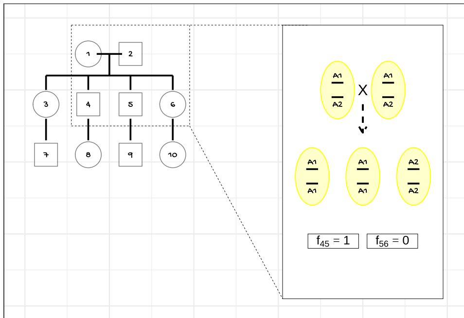
Figura 2.6: Parentesco observado entre individuos emparentados. El coeficiente de parentesco molecular entre los individuos 4 y 5, y 5 y 6, es igual a 1.0 y 0.0, respectivamente, caso contrario al coeficiente de parentesco genealógico, el cual entre todos los individuos, por tratarse de hermanos completos, sería igual a 0.25.
