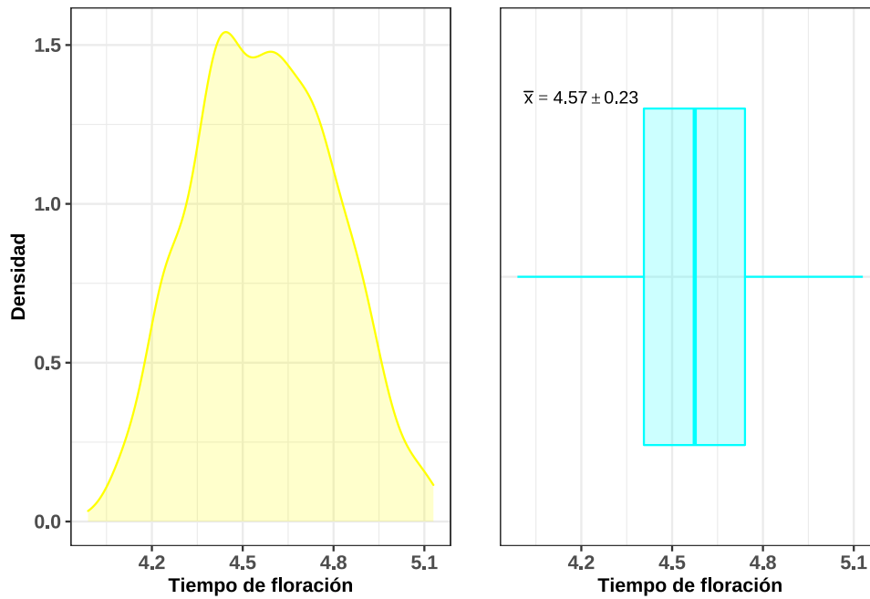
Figura 4.2: Distribución y media \pm desviación estándar del carácter tiempo de floración del conjunto de datos fenotípicos de arroz.
