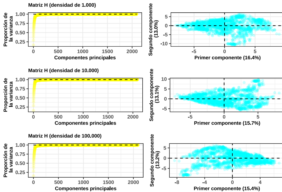
Figura 5.2: Análisis de componentes principales a partir de la matriz H resultante de la simulación de descendientes. Aquí, la matriz H se estimó a partir de 2091 individuos genotipados con densidad de marcador aproximada de 1.000, 10.000 y 100.000, y en el pedigrí 3 (primera réplica) mediante simulación de descendientes.
