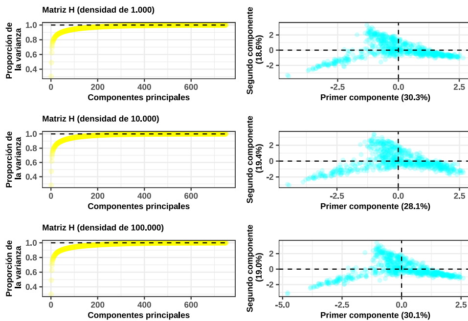
Figura 5.1: Análisis de componentes principales a partir de la matriz H resultante de la simulación ancestral. Aquí, la matriz H se estimó a partir de 451 individuos genotipados con densidad de marcador aproximada de 1.000, 10.000 y 100.000, y en el pedigrí 1 (primera réplica) mediante simulación ancestral.
