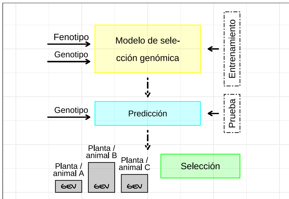
Figura 2.3: Esquema de la selección genómica. La selección genómica utiliza un modelo estadístico, diseñado a partir de datos genotípicos y fenotípicos en una población de entrenamiento, para predecir el GEBV de los individuos en una población de prueba con datos genotípicos. Por último, los individuos se seleccionan de acuerdo a su GEBV. Figura adaptada de Tong y Nikoloski (2021).
