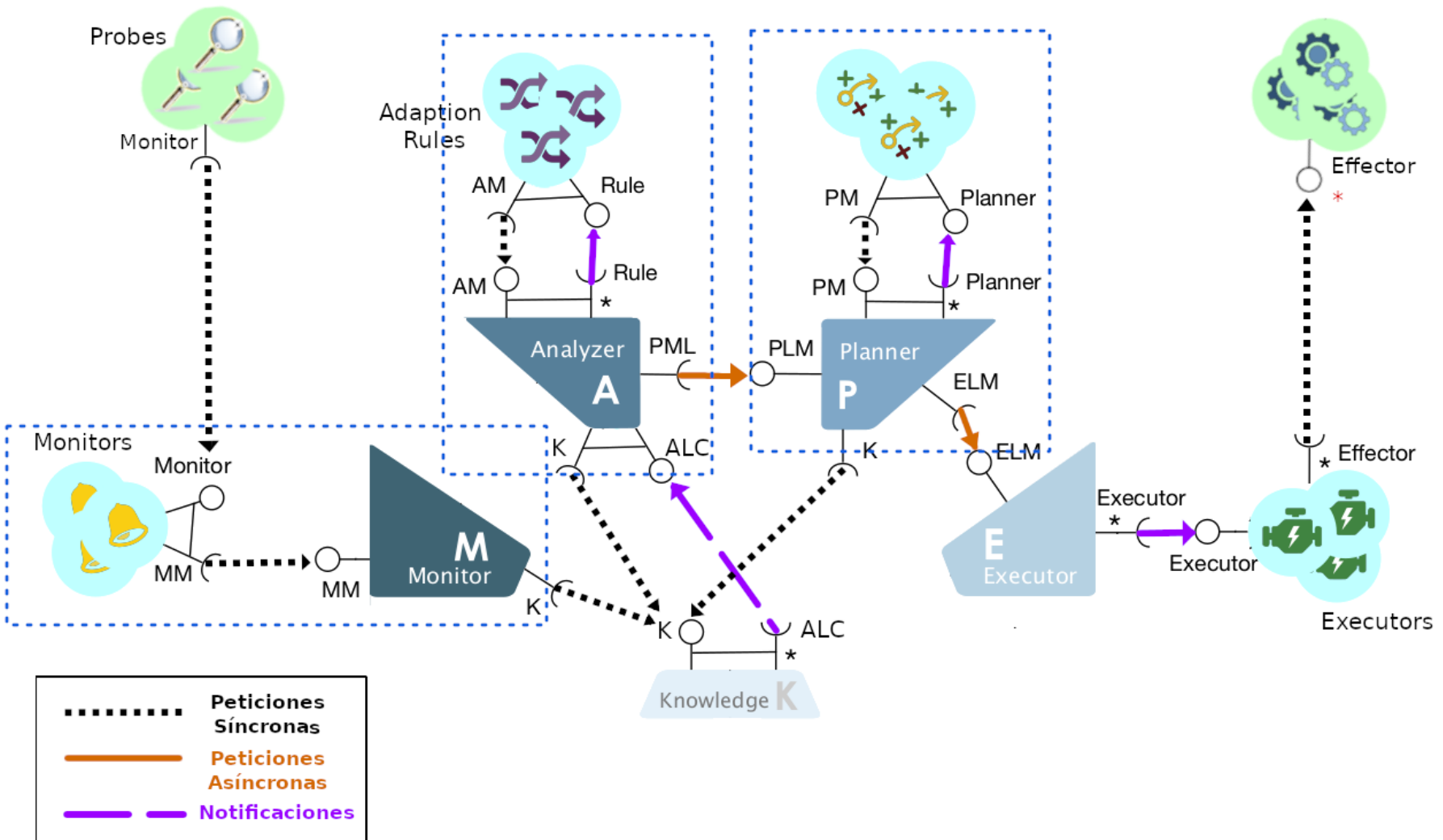
Figura 7.15: Propuesta arquitectónica final del bucle MAPE-K distribuido.
