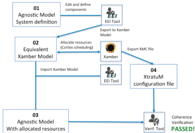
Figura 3 Flujo de trabajo IMA-SP
