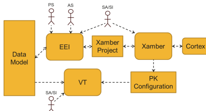
Figura 2 Arquitectura IMA-SP SDT
