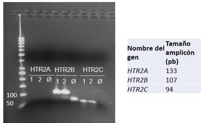
Figura B1. Electroforesis para comprobar los amplificados de la qPCR donde se testaron diferentes primers para marcadores neuronales en muestras de células neuroepiteliales. Se prepararon dos geles de agarosa al 3% y se empleó un marcador de pesos moleculares de 50 pb (Thermofisher). Para cada gen se testaron dos réplicas (1 y 2). Como control negativo se empleó agua (Ø). Para cada gen se indica su correspondiente tamaño de amplicón (pb).
