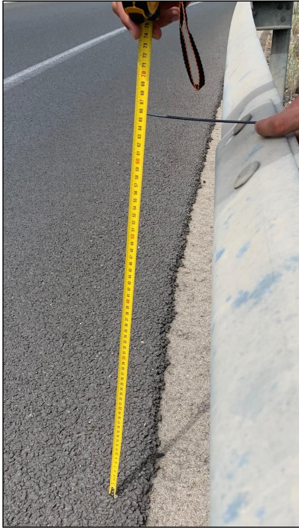
Figura 13. Altura de la barrera metálica en el PK 3+050 ascendente.
