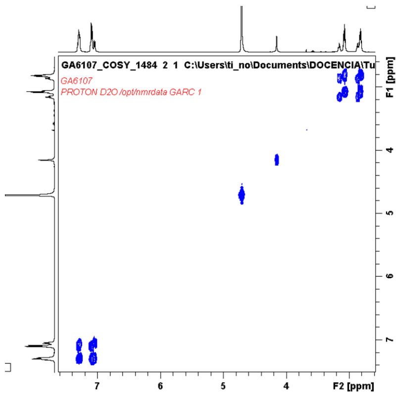
Espectro COSY de TPA-Tren en D 2 O.
