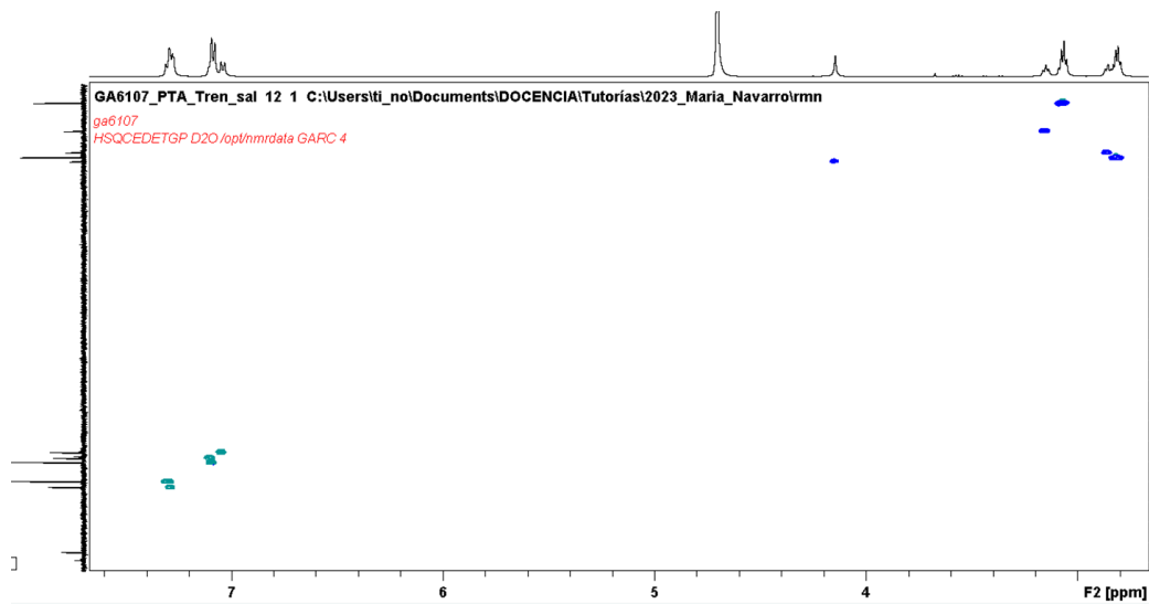
Espectro HSQC de TPA-Tren en D 2 O.
