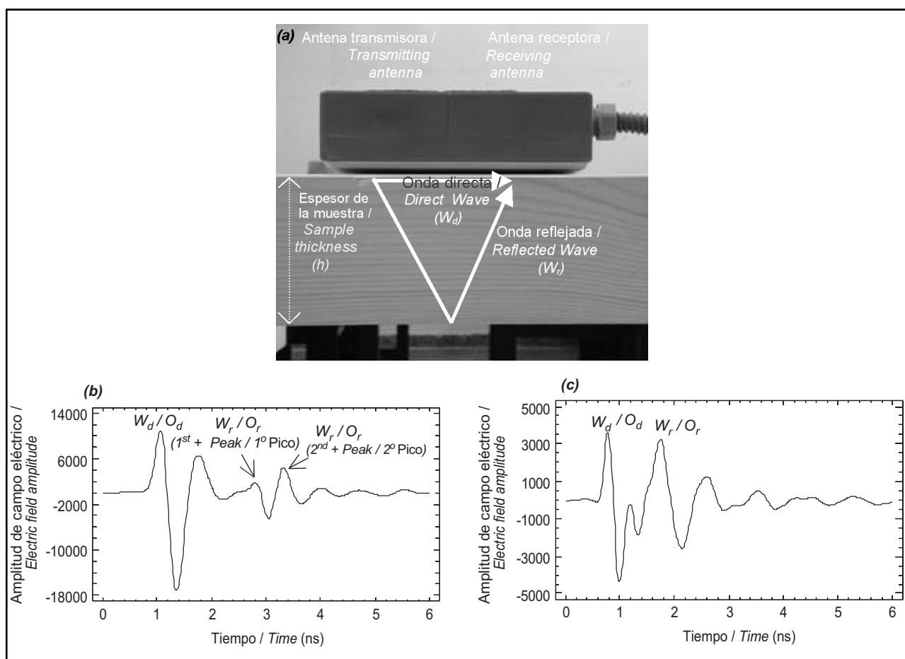
Figura 3. (a) Recorrido de la onda directa y reflejada; (b) Señal característica registrada al atravesar el lado A; (c) Señal característica registrada al atravesar el lado B.
