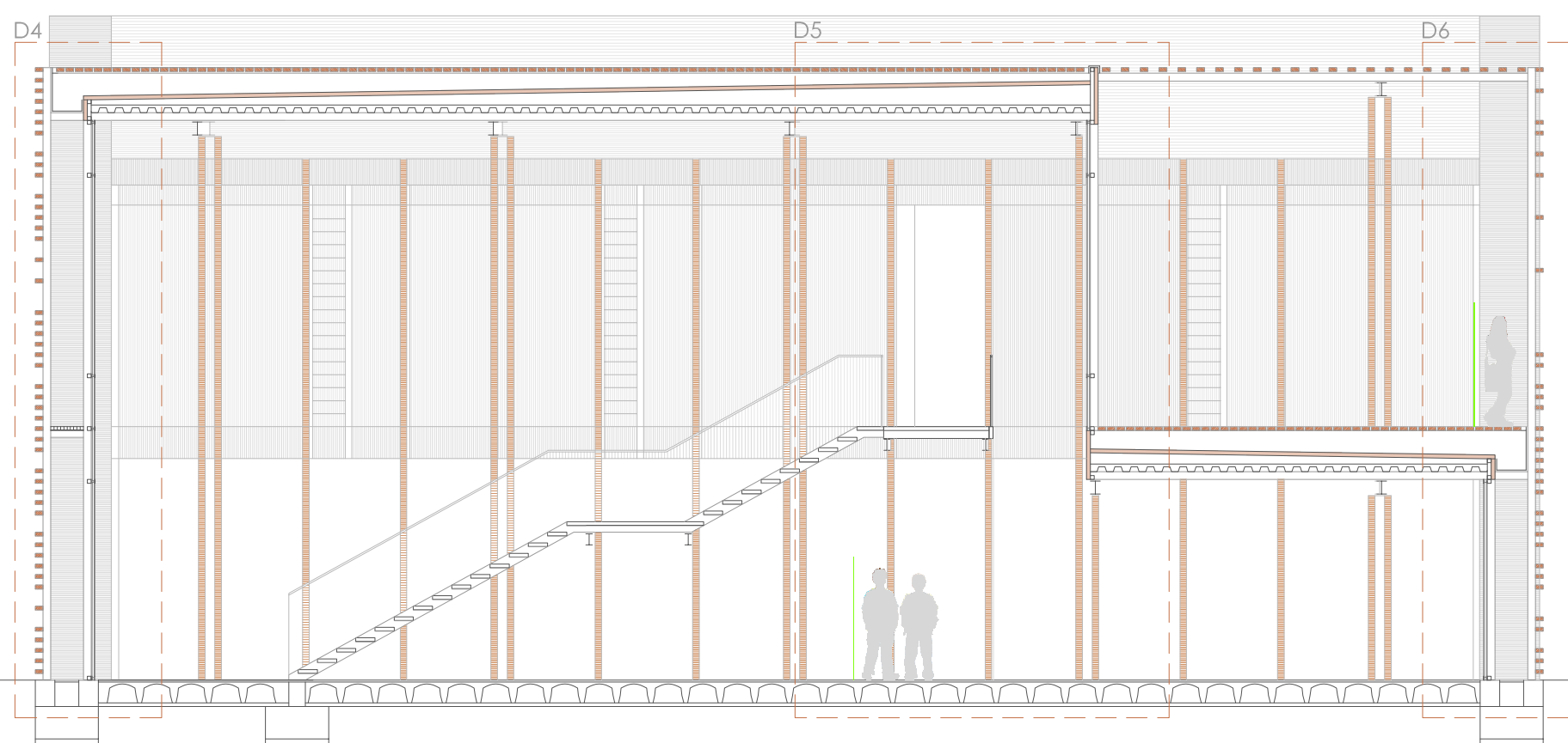
Sección B/ escala 1:100
