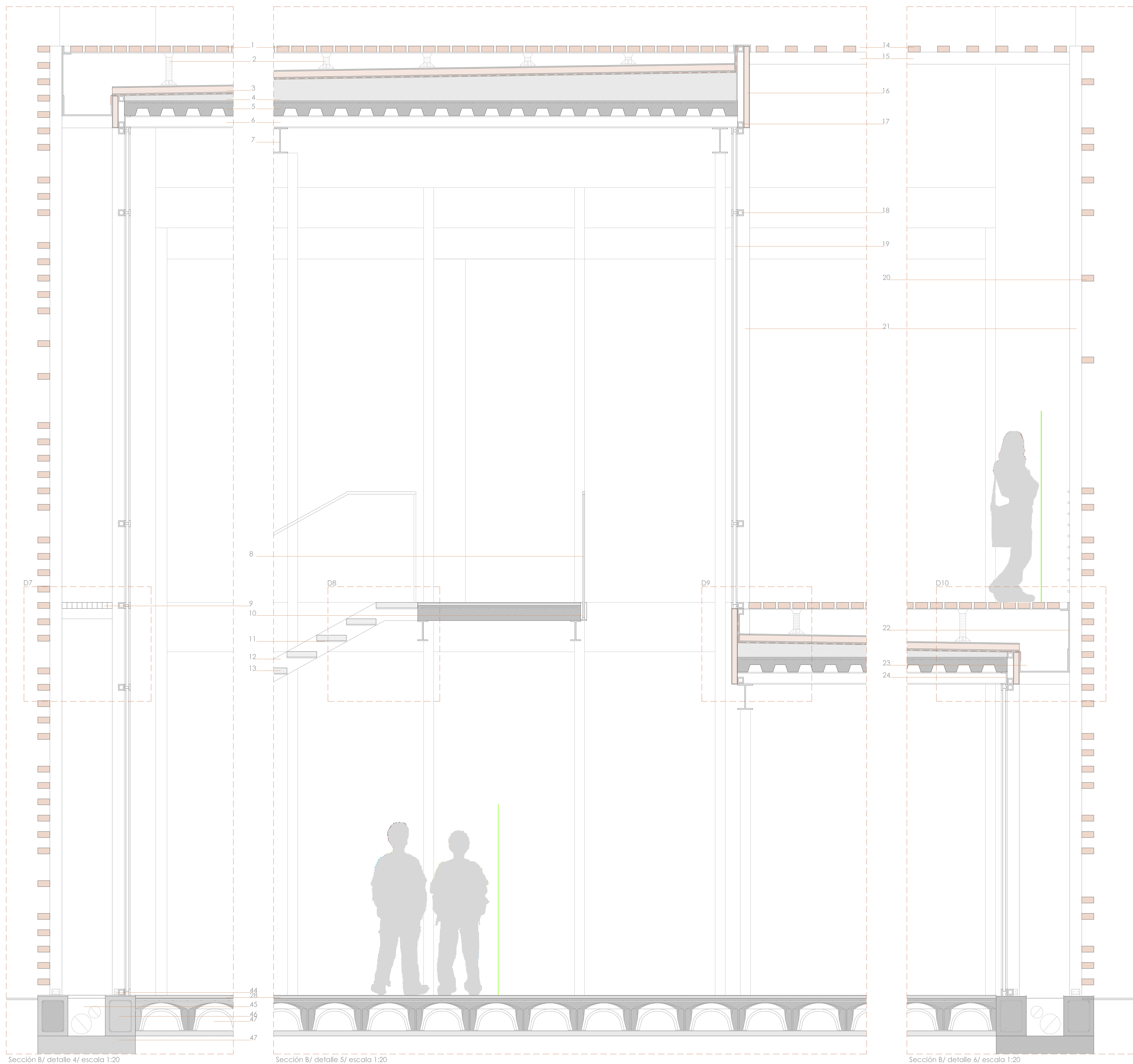
Sección B/ detalle 4/ escala 1:20
