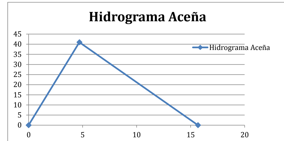
Ilustración 9. Hidrograma unitario Rambla Aceña.
