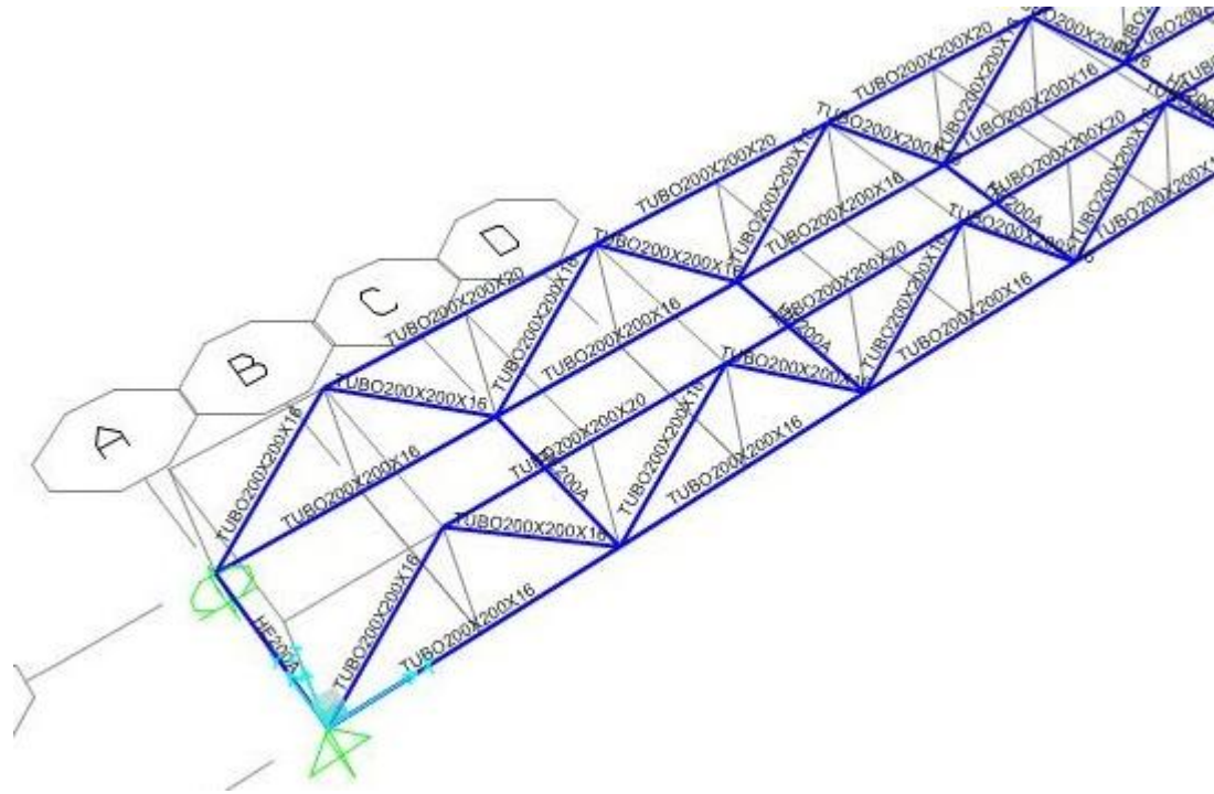
Ilustración 3: Cercha
