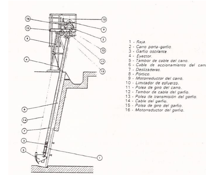
Ilustración 1. Reja con dispositivo automático de limpieza
