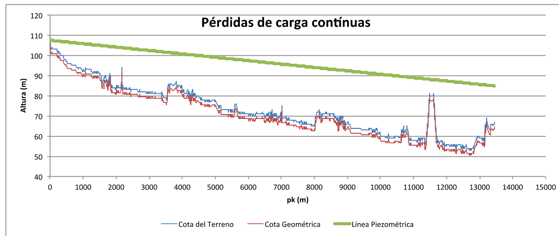
Gráfico 1. Pérdidas de carga continuas. Piezométrica.
