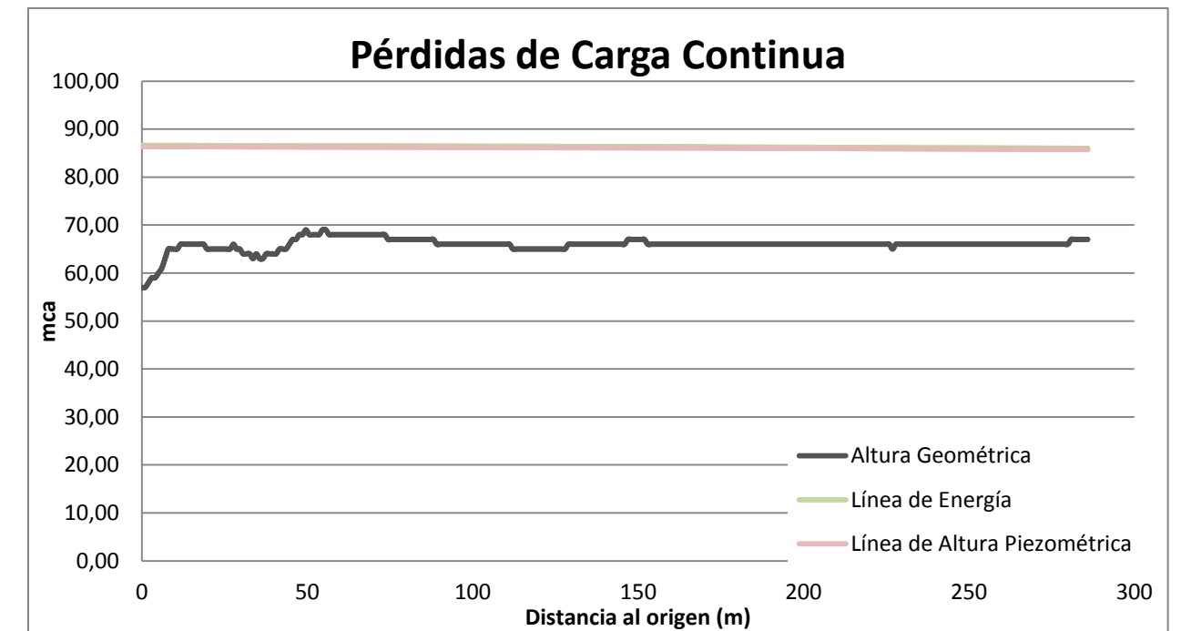
Figura 3: Gráfico Pérdidas Continuas, Cámara de Reparto 3.
