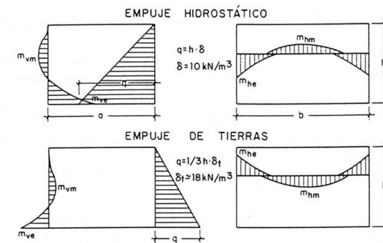
Ilustración 1. Leyes de momentos flectores
