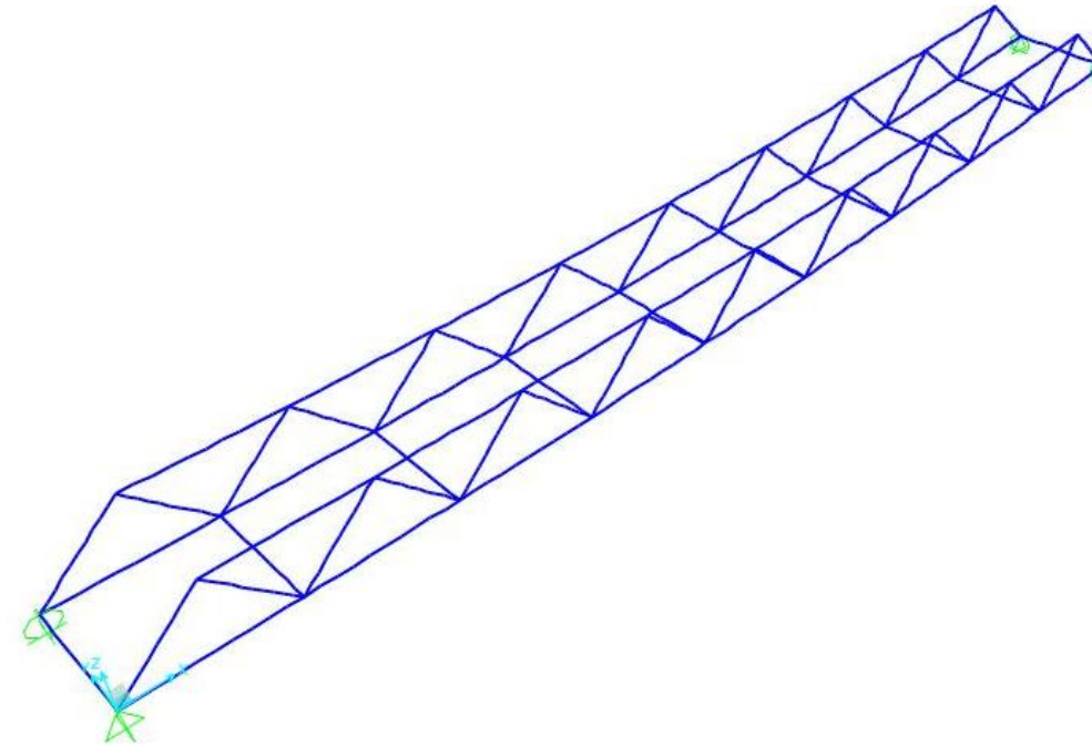
Figura 11: Deformada (Flecha máx. ELS: 0.119 m)
