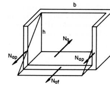
Ilustración 7. Esfuerzos de tracción.
