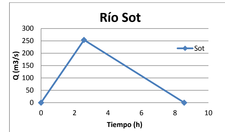
Ilustración 7. Hidrograma unitario Río Sot. Captación 1
