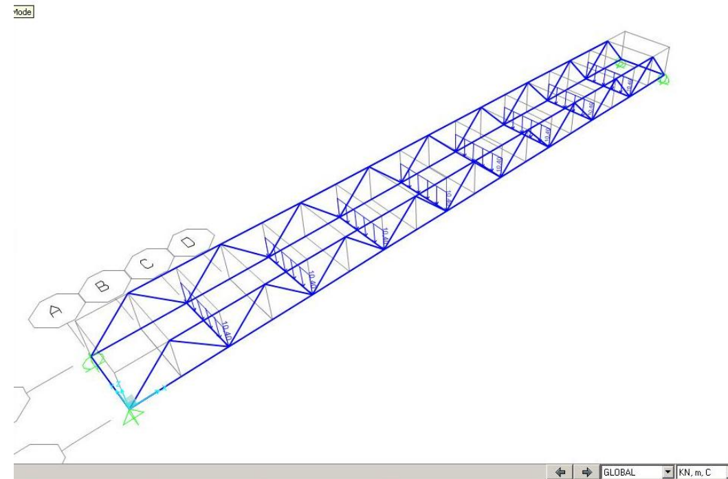
Figura 4: Peso Propio
