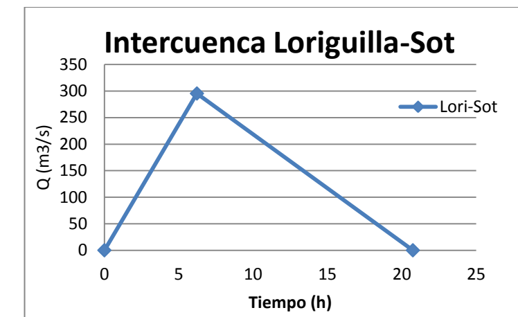
Ilustración 8. Hidrograma unitario Intercuencia Loriguilla-Sot. Captación 1
