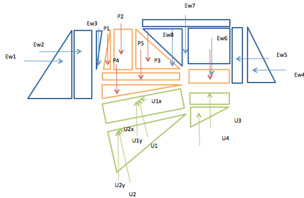
Ilustración 3. Fuerzas resultantes
