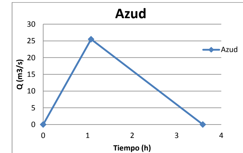
Ilustración 12. Hidrograma unitario Subcuenca Azud. Captación 1
