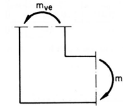
Ilustración 8. Momentos de empotramiento pared-solera: m_{ae} = m_{ve}
