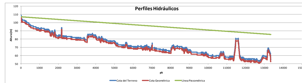
Ilustración 9. Línea de alturas piezométricas. Tubería. C1.
