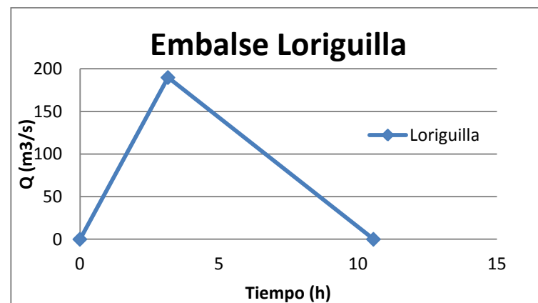
Ilustración 6. Hidrograma unitario embalse Loriguilla. Captación 1
