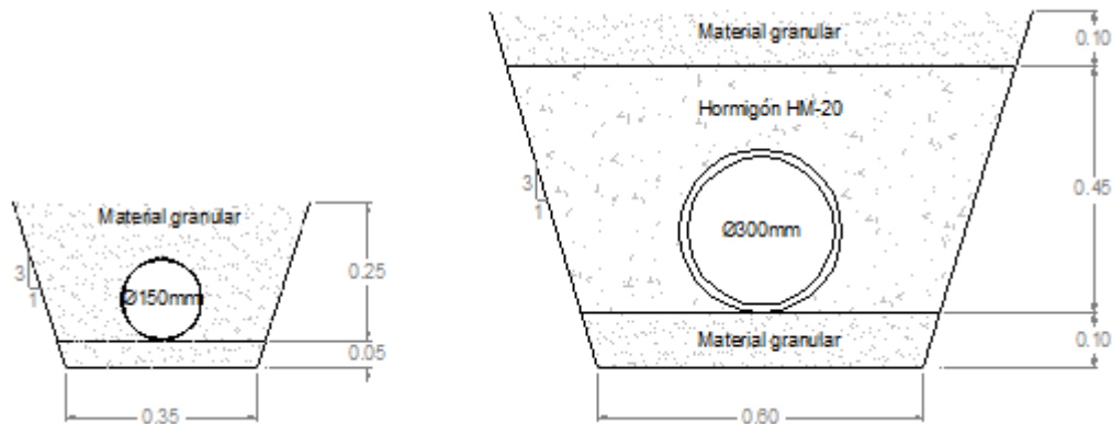
Figura VII.1. Zanjas de 150 mm y 300mm de diámetro.
