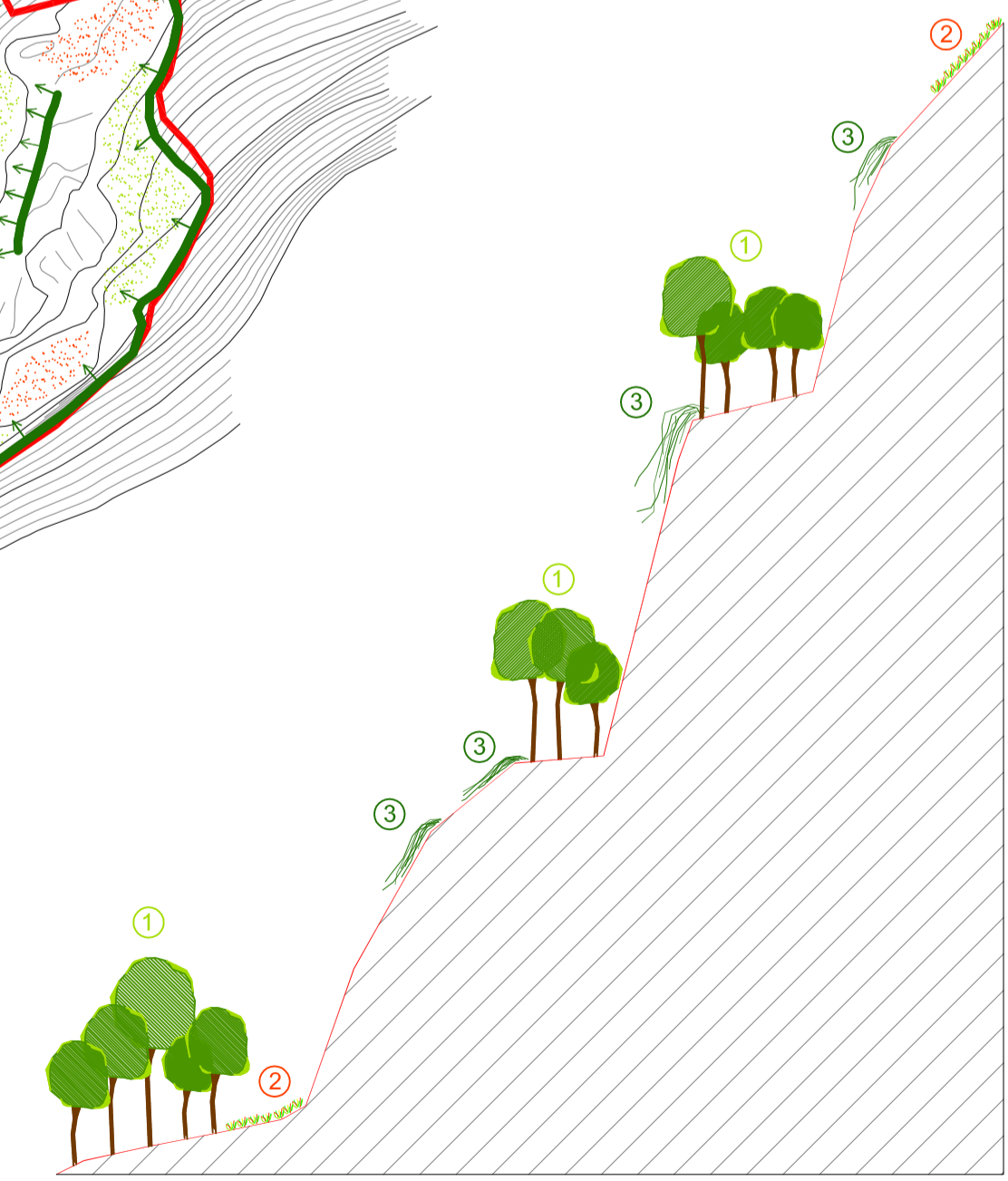
DETALLE PLANTACIONES PERFIL TIPO ESCALA 1/500
