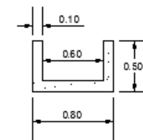
Cuneta tipo 3
