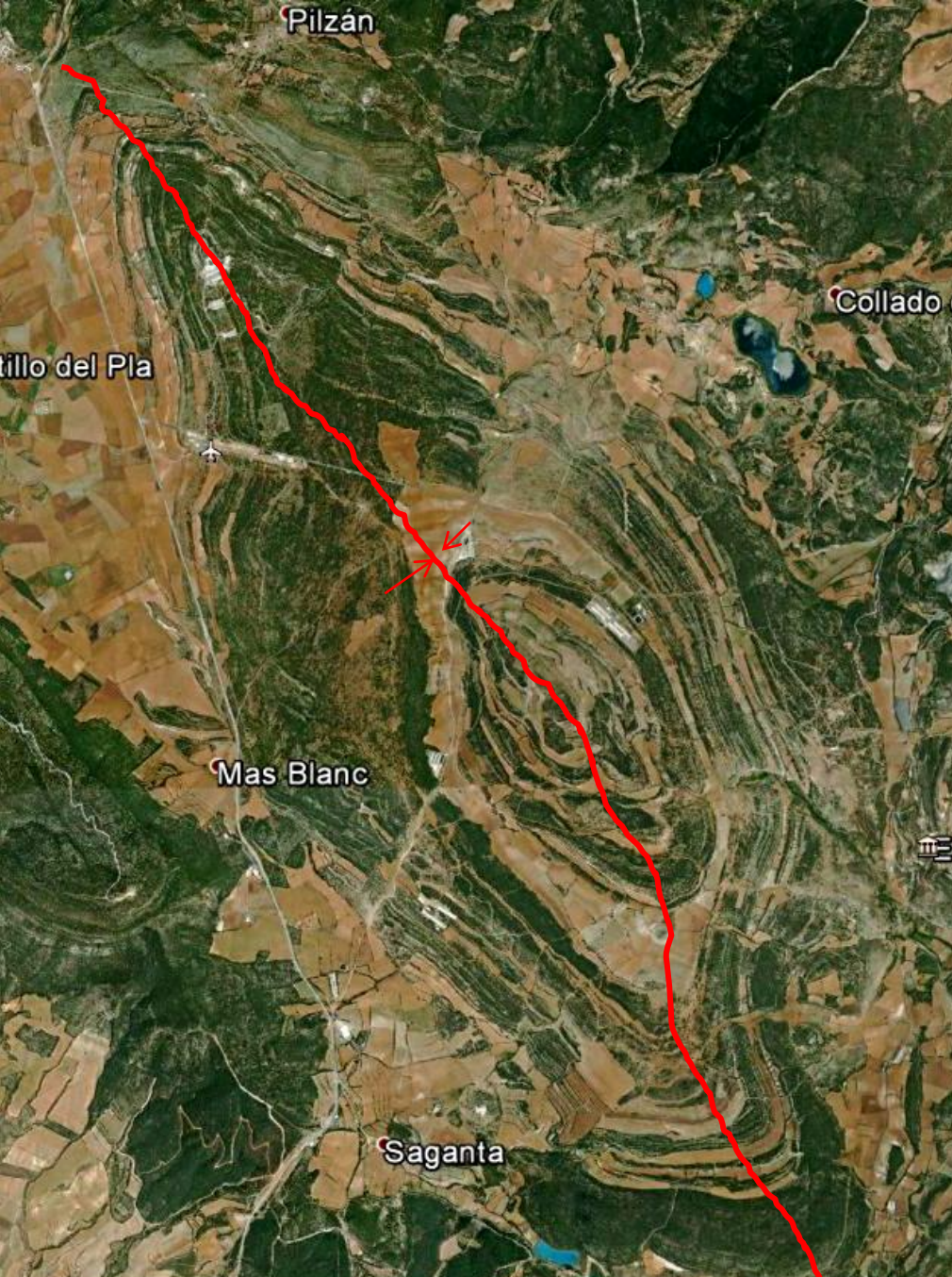
Sinclinal en materiales del Eoceno, Terciario. SW Hoja de Benabarre- NW de la de Os de Bañaguer. Perspectiva – relieve realizado-desde el SW.
