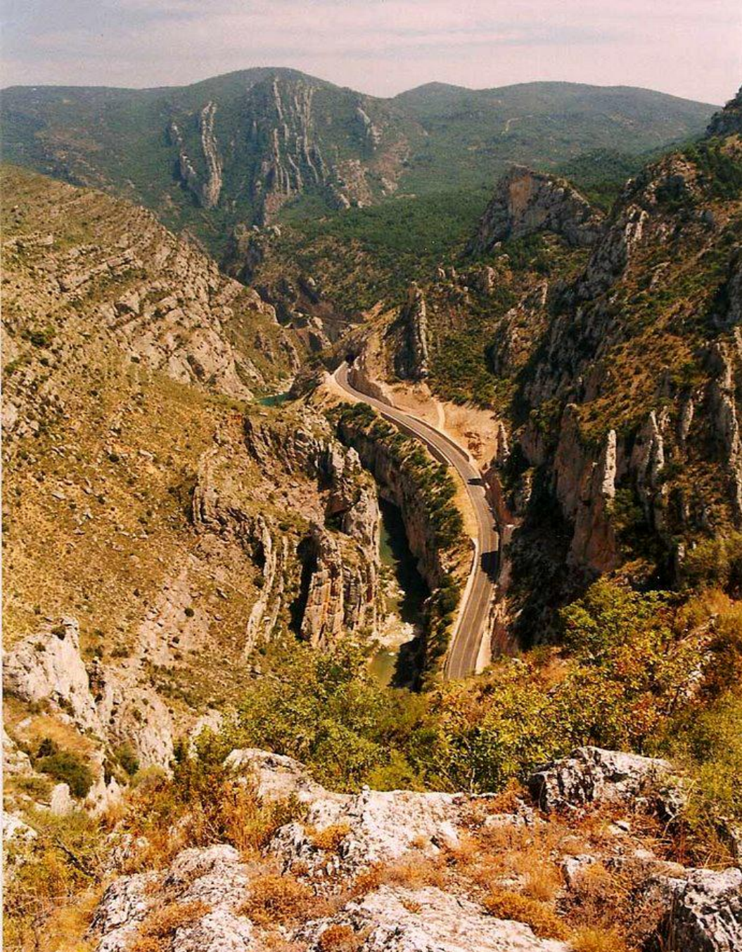
Calizas del Cretácico Sup., subverticales. Congosto de Olvena, Huesca. Y detalle. Centro NW Hoja de Fonz. (por carlos portoles/monegros 042008-google)
