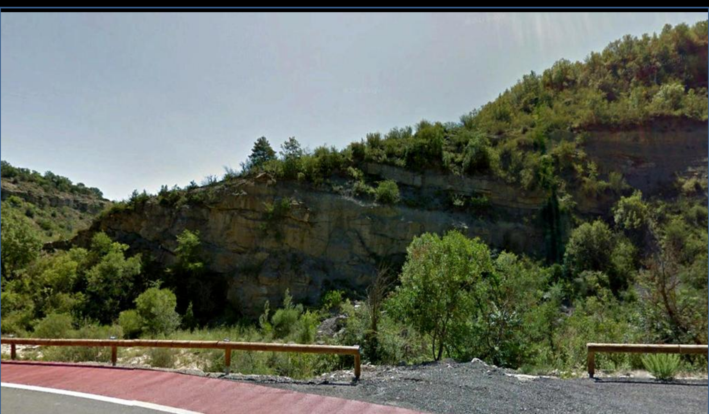
Areniscas y lutitas del Cuisiense, Eoceno, Terciario. E de Montañana, Huesca. N Centro E Hoja de Benabarre.
