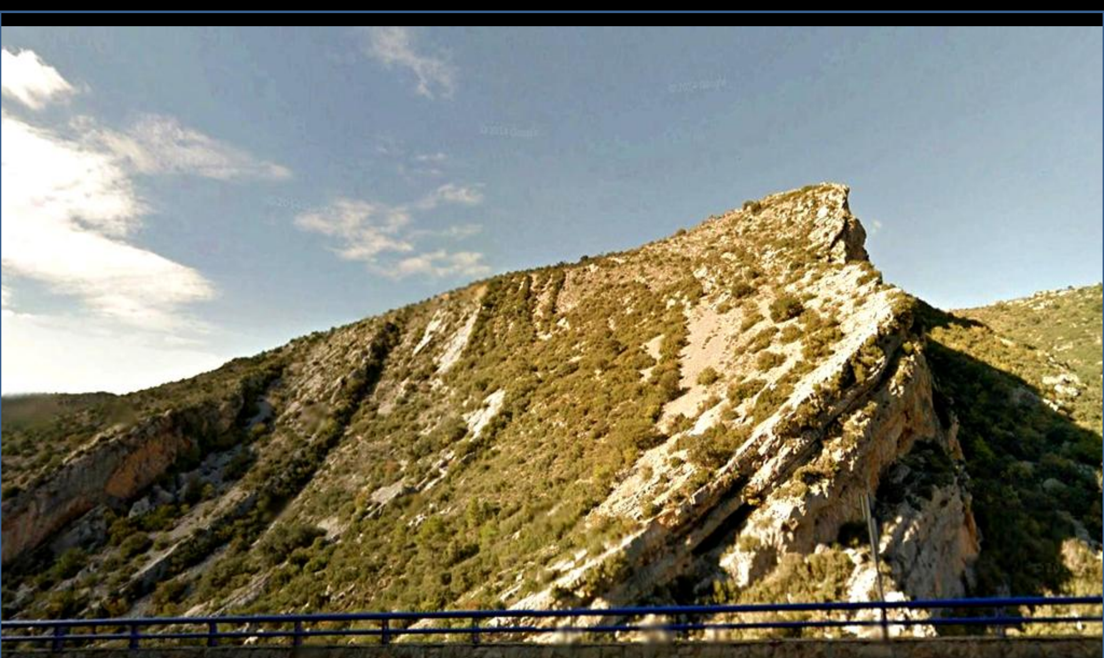
Calizas del Cretácico Sup. Congosto de Olvena, Río Esera. La Puebla de Castro, SW del Embalse de Barasona. Huesca. Centro NE Hoja de Fonz.
