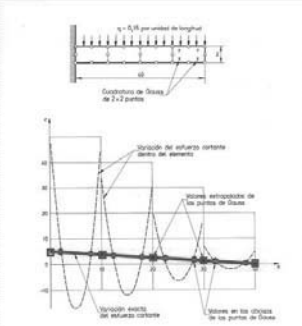
Figura 5.25 Viga en voladizo analizada con cuatro elementos Serendipíticos de 8 nodos. Valores del esfuerzo cortante en las secciones correspondientes a la cuadratura \int_{-1}^1 de Gauss-Legendre y correspondencia lineal a los nodos.
