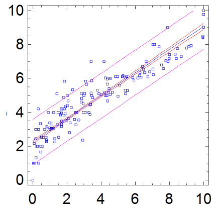
Gráfico 10. Gráfico de la regresión entre TrustRank y PageRank
