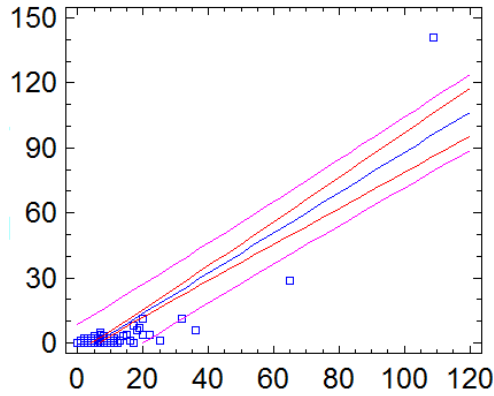
Gráfico 17. Gráfico de la regresión entre Me_Gusta y Veces_Compartido
