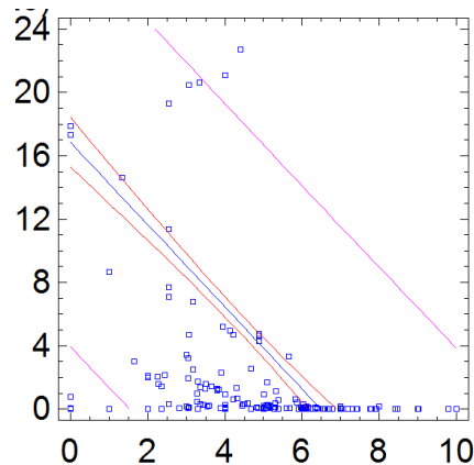
Gráfico 11. Gráfico de la regresión entre el PageRank y el Ranking en Alexa
