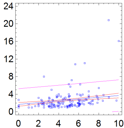
Gráfico 9. Gráfico de la regresión entre el PageRank y Páginas por visitante_día
