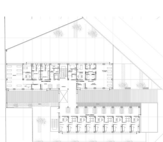
PLANTA PRIMERA
