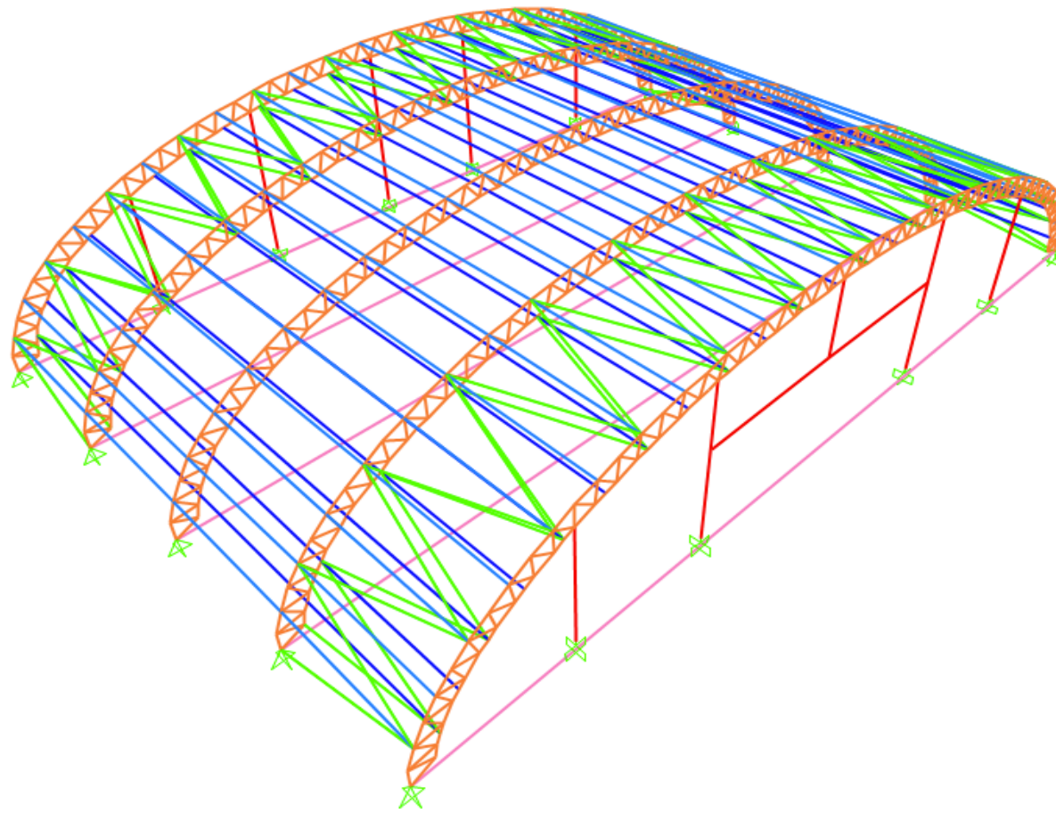
Figura 3.a Visión general estructura. Captura Sap2000.
