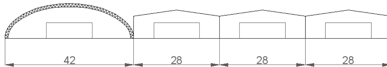
Figura 2. Definición geométrica infraestructuras. Captura AutoCad.
