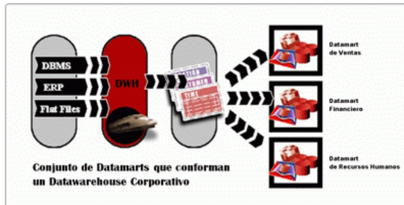
Ilustración 14: Proceso ETL
