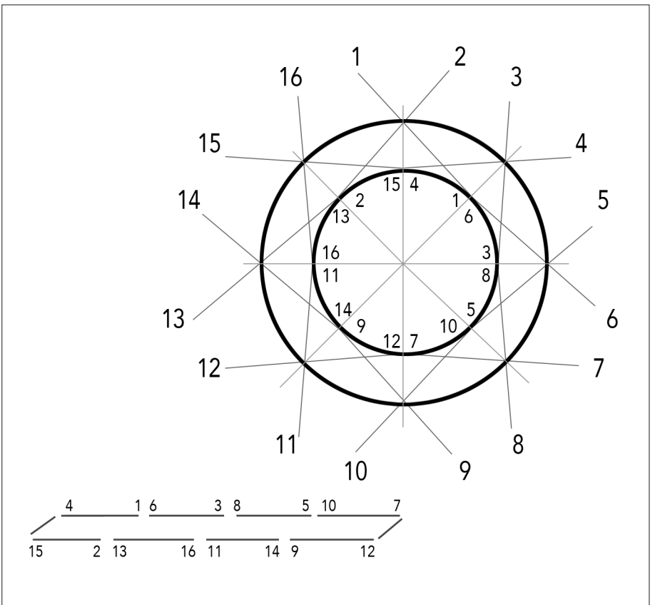
Esquema de relacions òptiques
