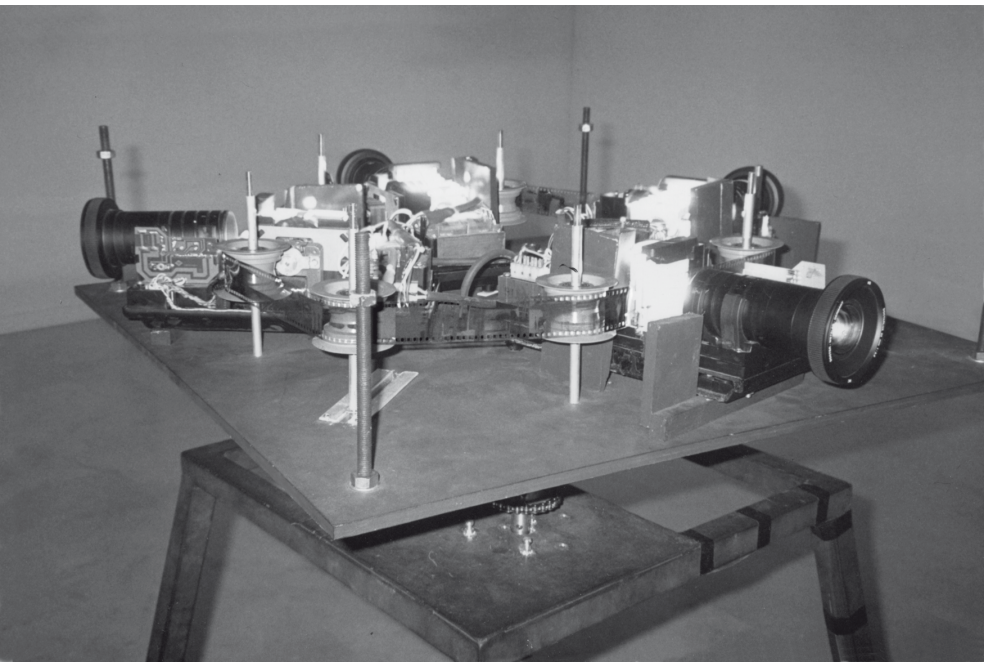
Maquinària de multiprojecció: projectors rectificats, rodets, motors i engranatges
