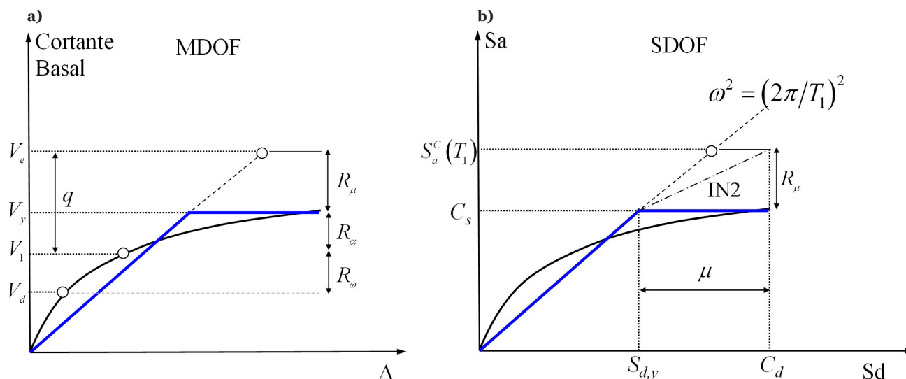
Figura 1. CC idealizada para una estructura desnuda (a) y en formato ADRS con su correspondiente IN2 (b).
