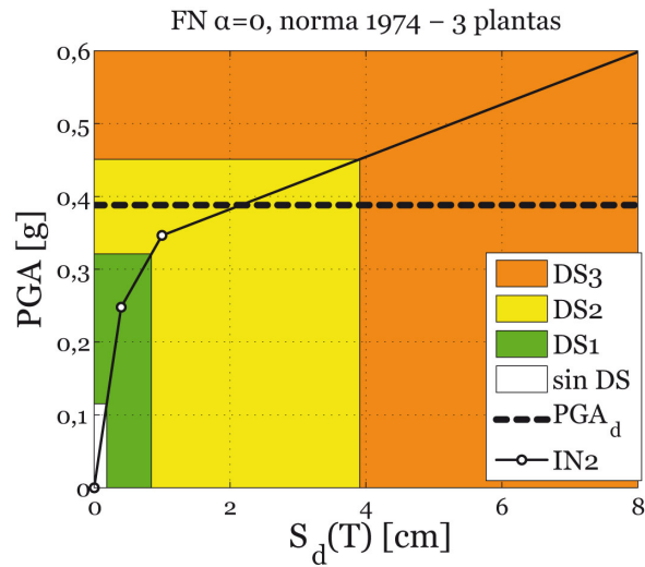
Figura 11. Daño medio esperado para edificios de 3 plantas según PDS-1 para la dirección FN, sin contribución del HA antes de la degradación de la tabiquería.
