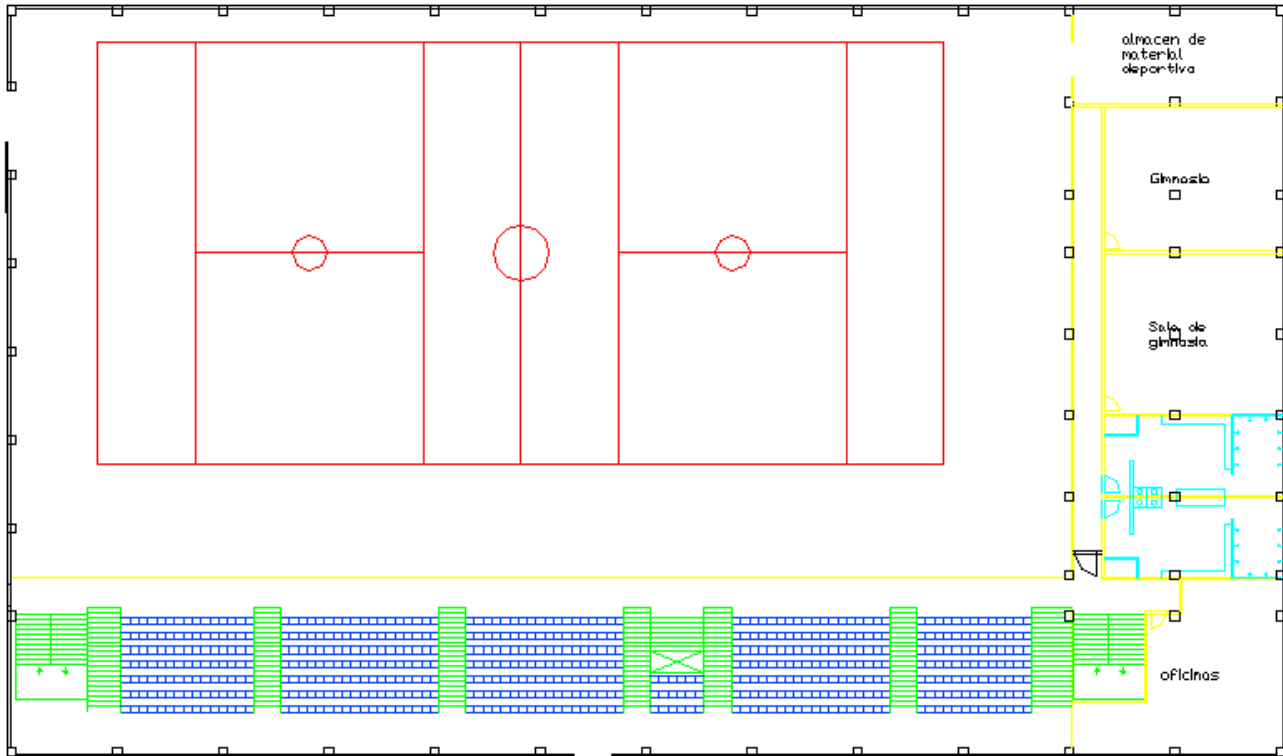
Figura 5 : Distribución de la segunda planta
