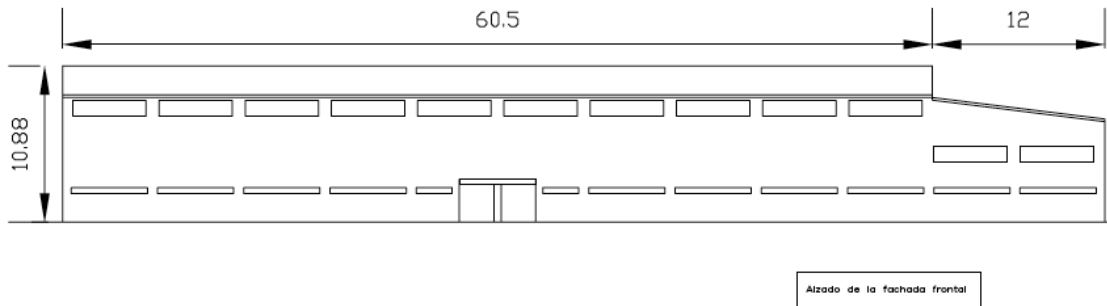
Alzado de la fachada frontal Figura 10 : Fachada principal con ventanas
