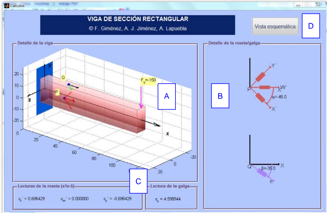
Fig. 3. Ejemplo de uso: lecturas de las microdeformaciones de la galga y de la roseta
