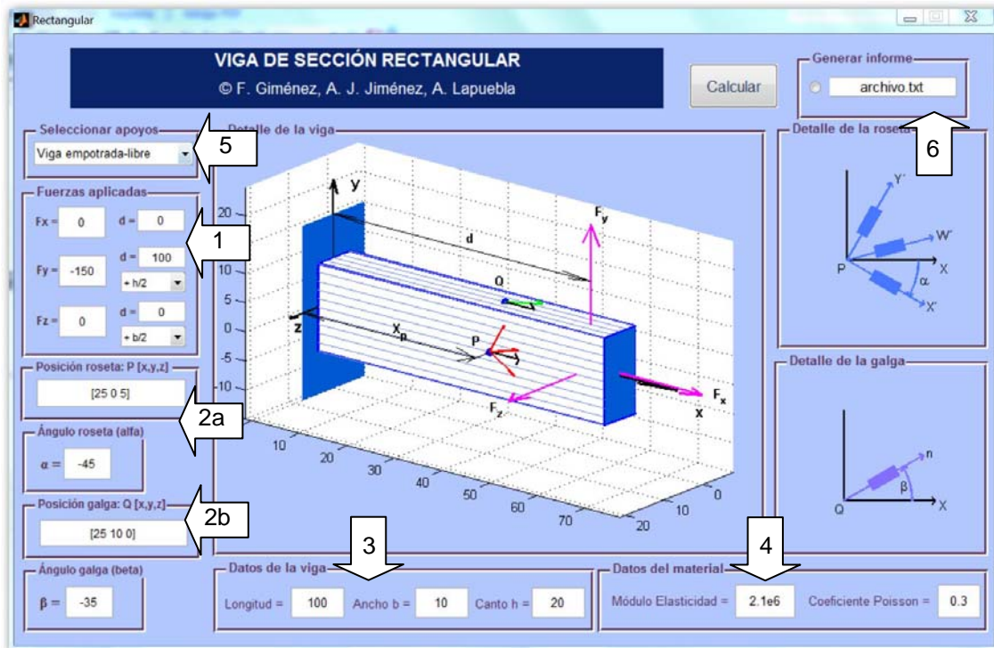
Fig. 1. Interfaz de usuario del laboratorio virtual RECTANGULAR
