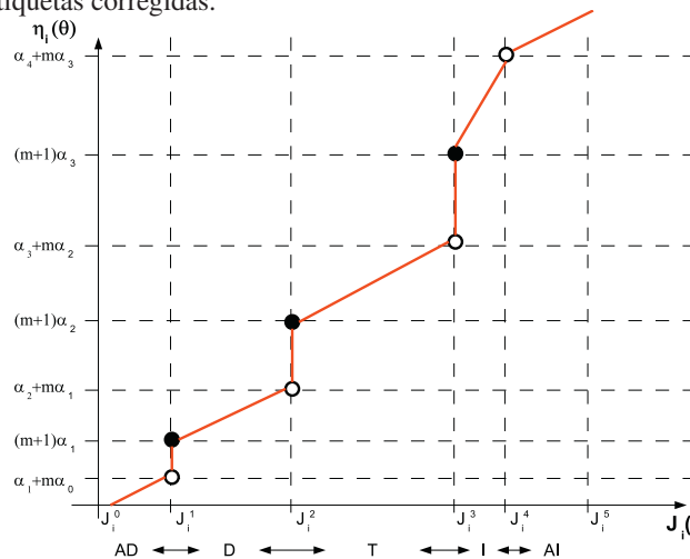
Figura 7: Función de clase propuesta.
