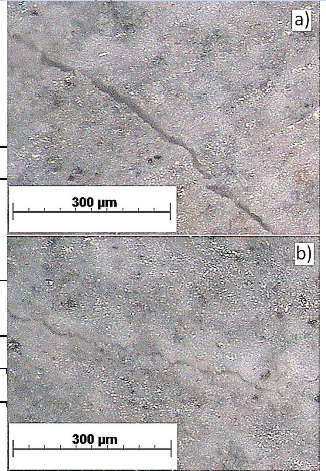
Figura 1. Fisura sobre las pastas de cemento con fibras, a) PP y b) PVA. Fuente: Elaboración propia, 2011.
