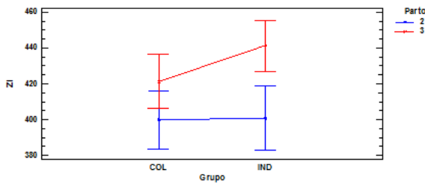
Figura 8.- Comparación entre la jaula colectiva (COL) e individual (IND) sobre la ingestión de las conejas (ZI) en el parto 2 y 3.
