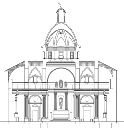
Sección transversal
