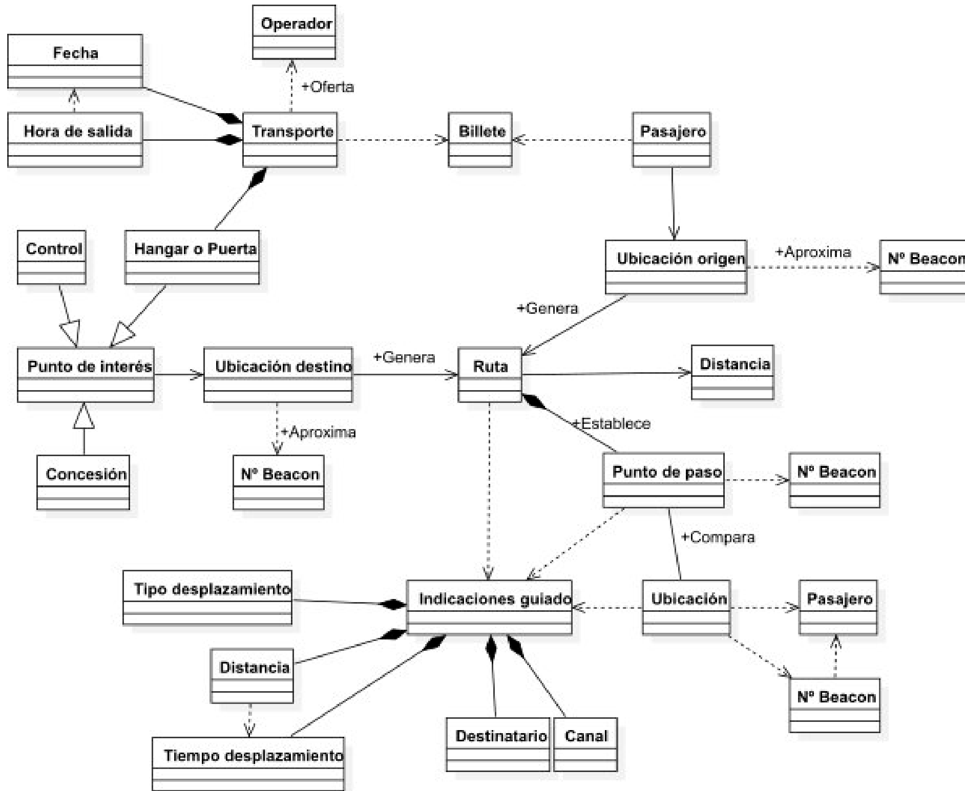
Diagrama de clases: Posicionamiento y guiado (Figura 15)
