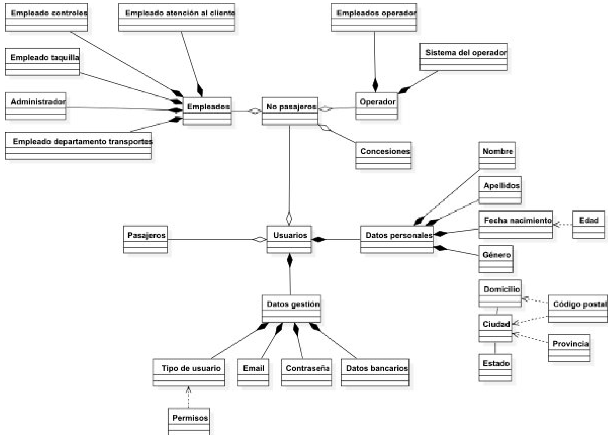
Diagrama de clases: Datos de usuario (Figura 12)
