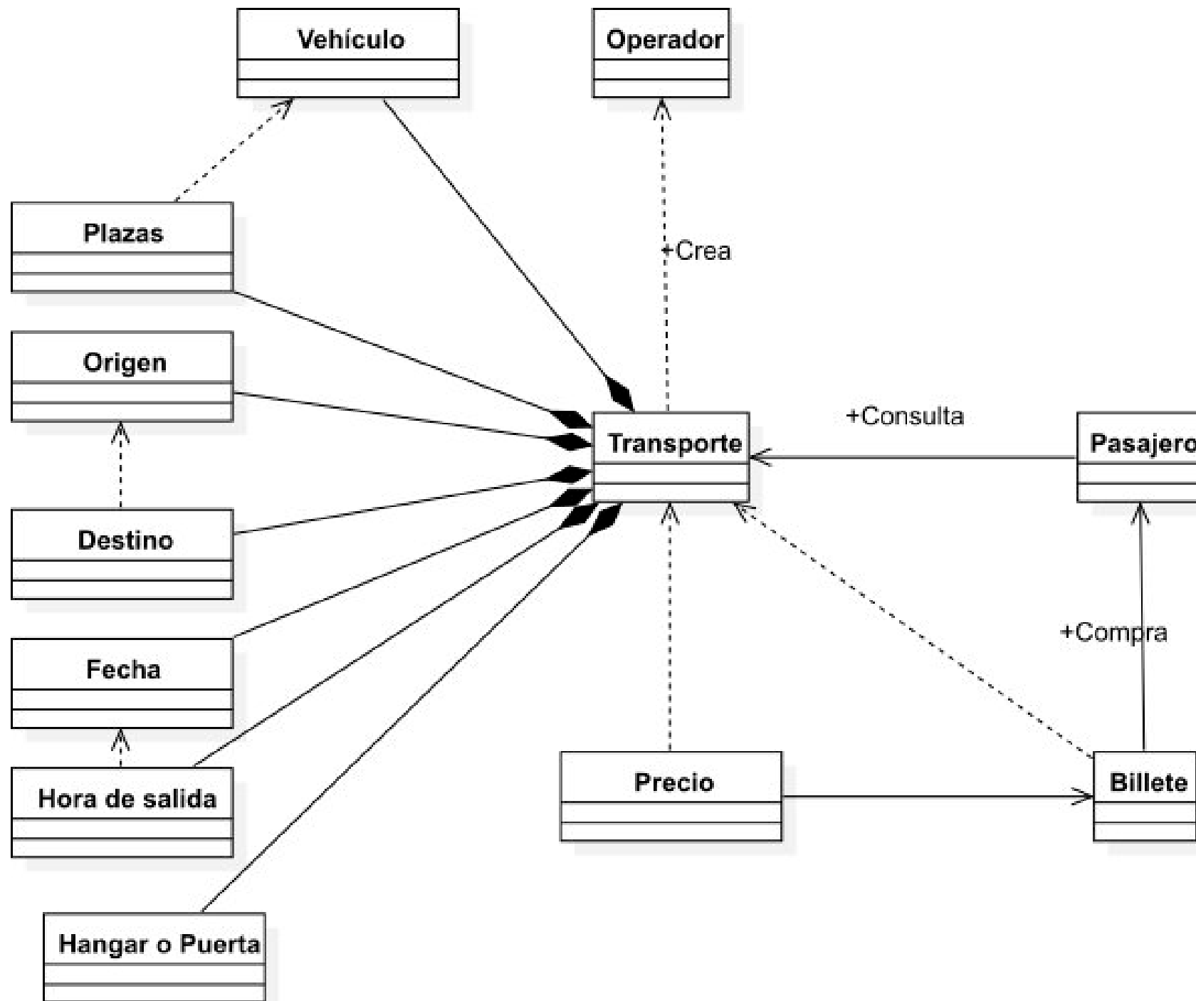
Diagrama de clases: Gestión de la oferta y compra de billetes (Figura 13)
