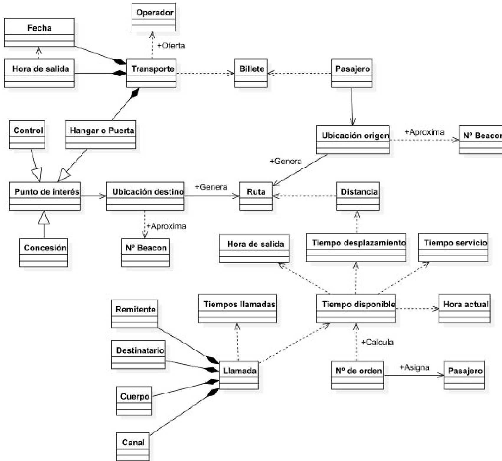
Diagrama de clases: Secuenciación y llamada de usuarios (Figura 14)
