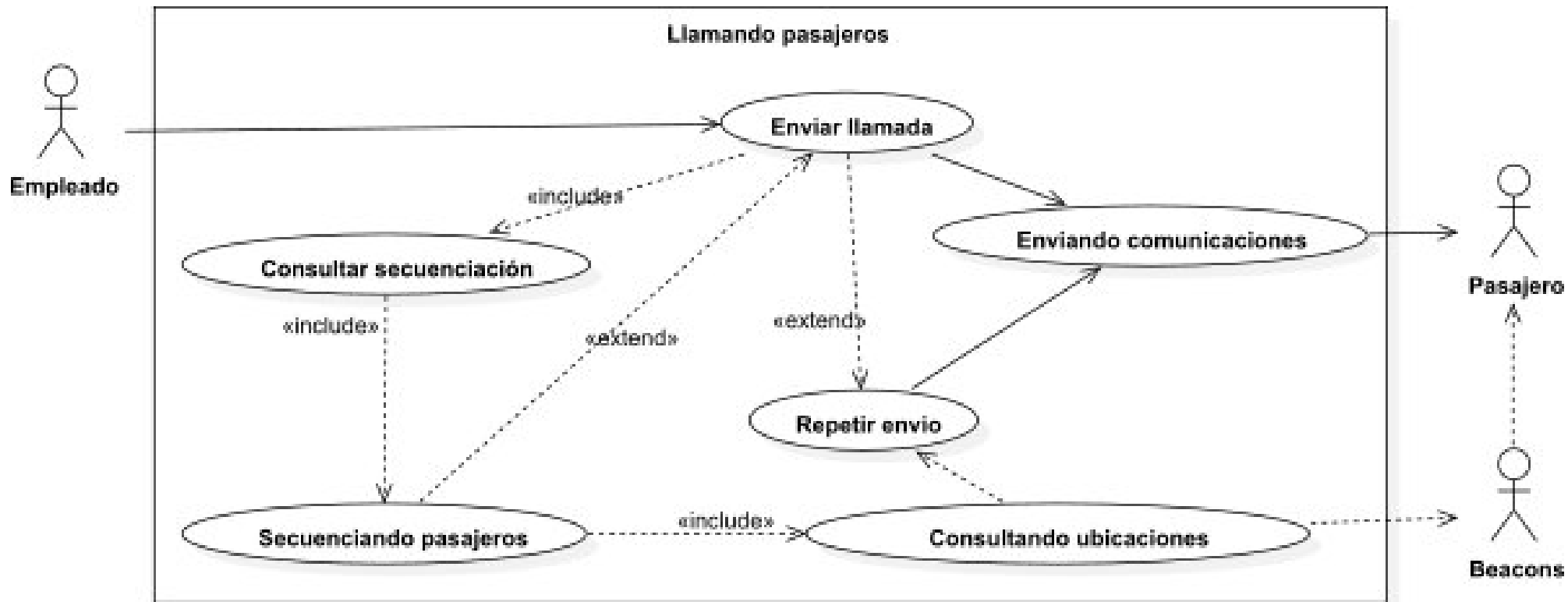
Caso de uso: Llamando pasajeros
