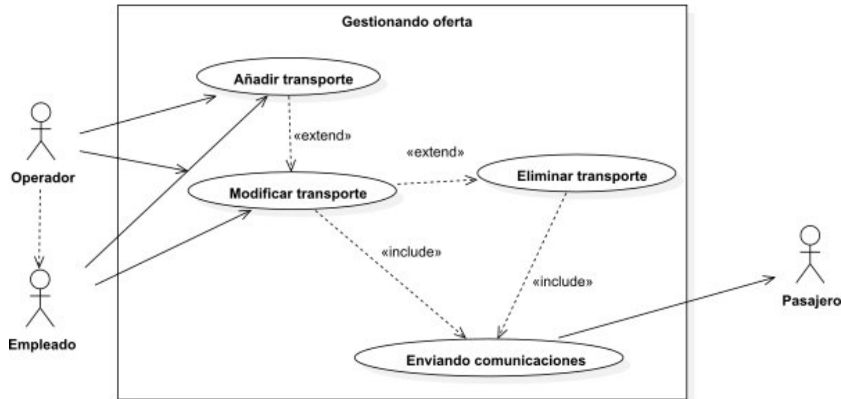
Caso de uso: Gestionando oferta
