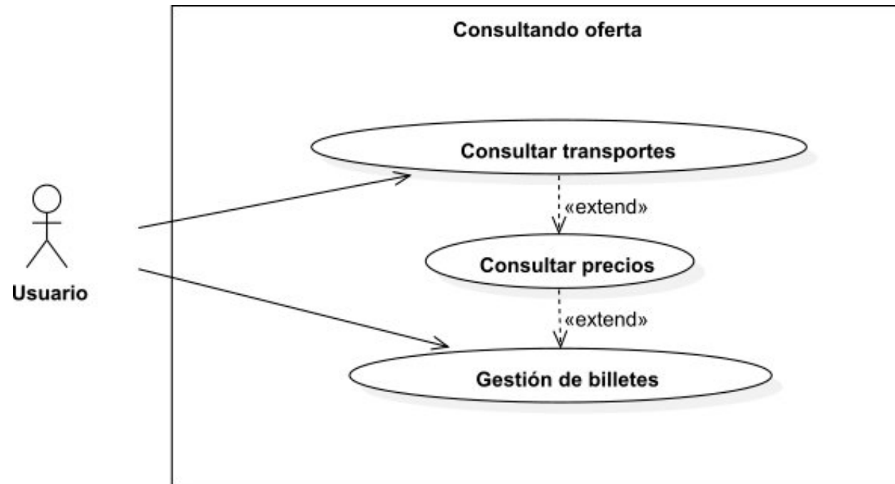
Caso de uso: Consultando oferta
