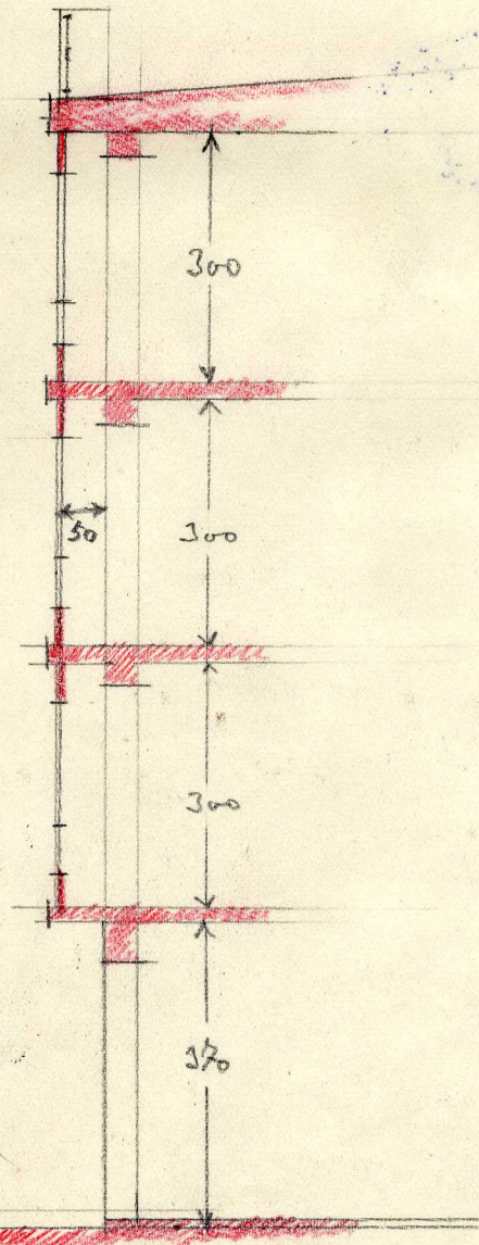
SECCION S1'
