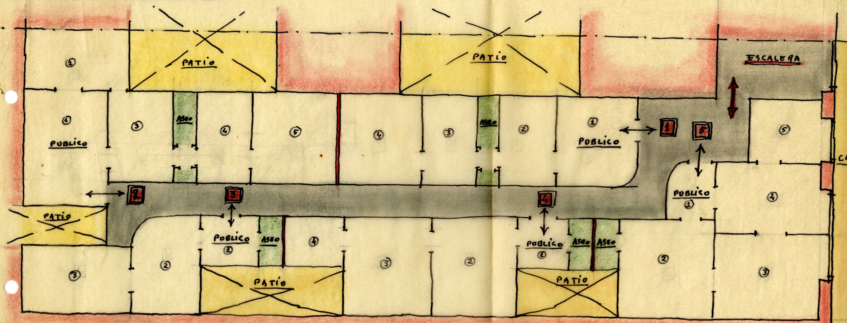
SOLUCION DE CINCO DESPACHOS E. - 1:100
