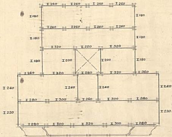
Planta 2º piso
