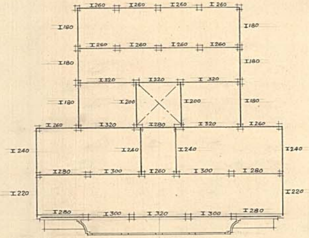
Planta 5º y 6º
