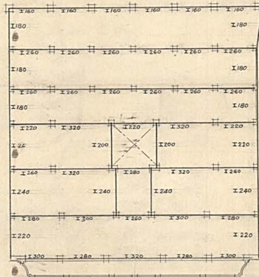
Planta del 1º piso
