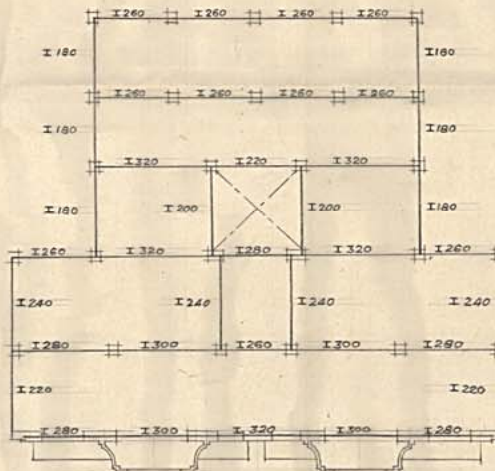
Planta 3ª y 4ª piso
