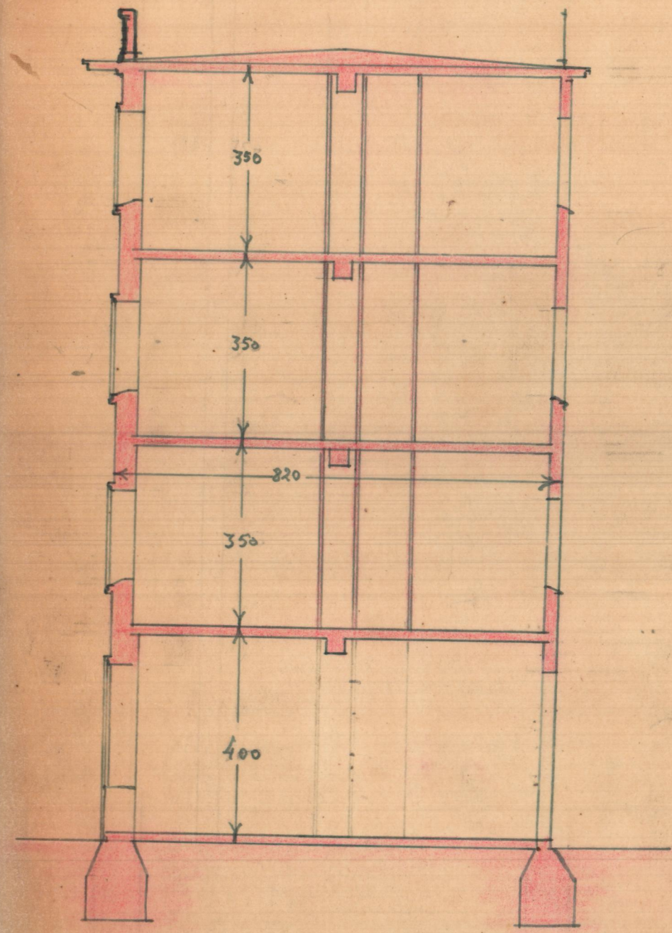
SECCION AB
