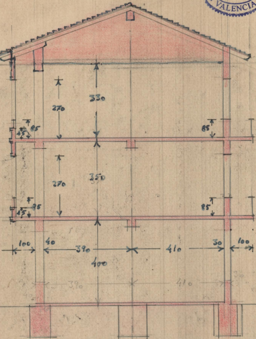
SECCION TRANSVERSAL
