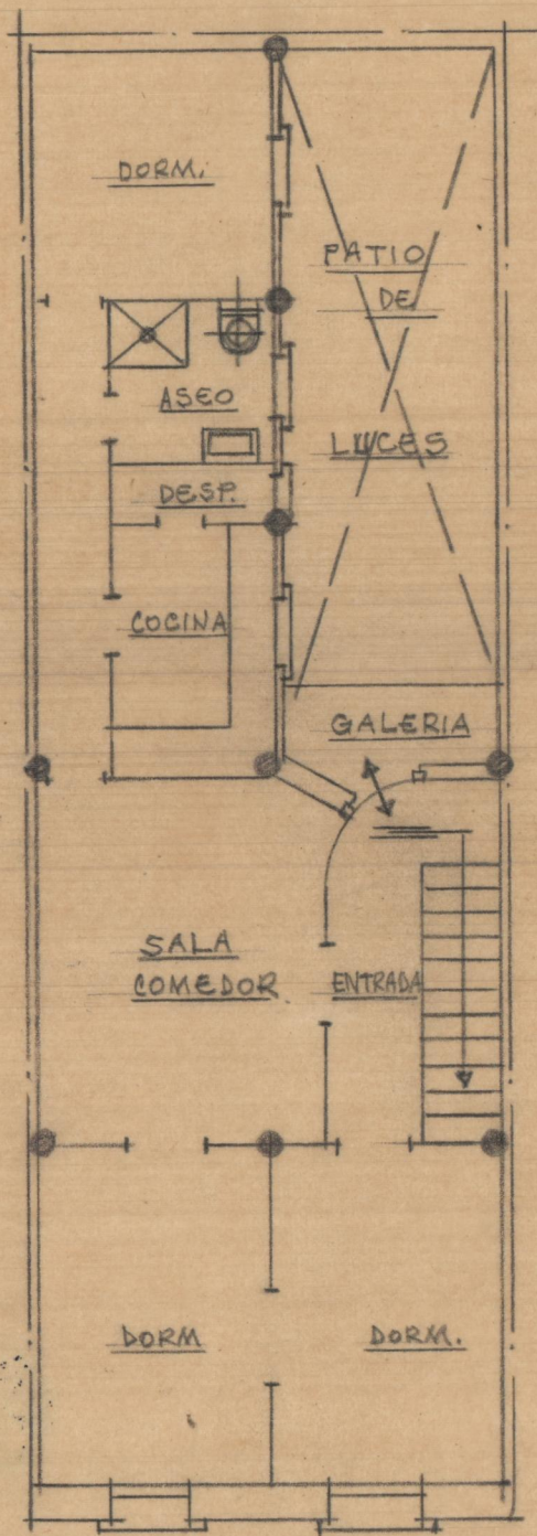
Croquis de disposici3n E=1:100
