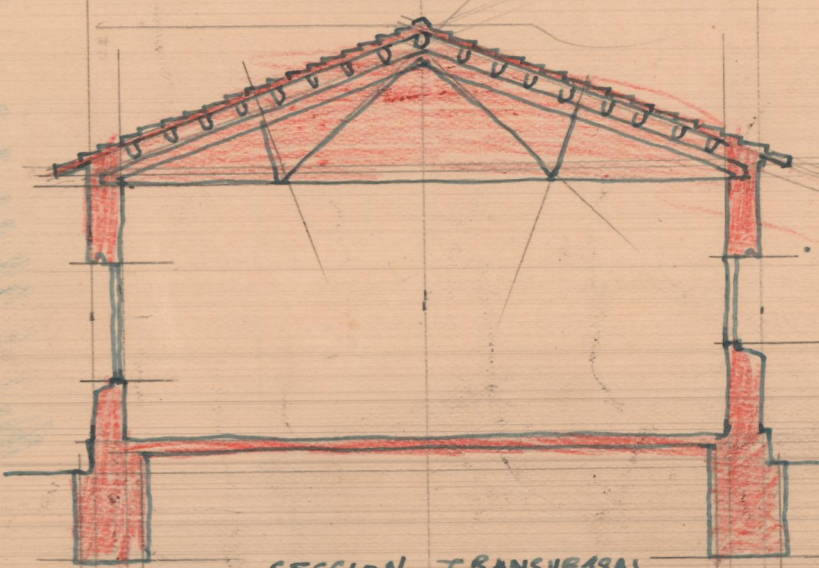
SECCION TRANSVERSAL
