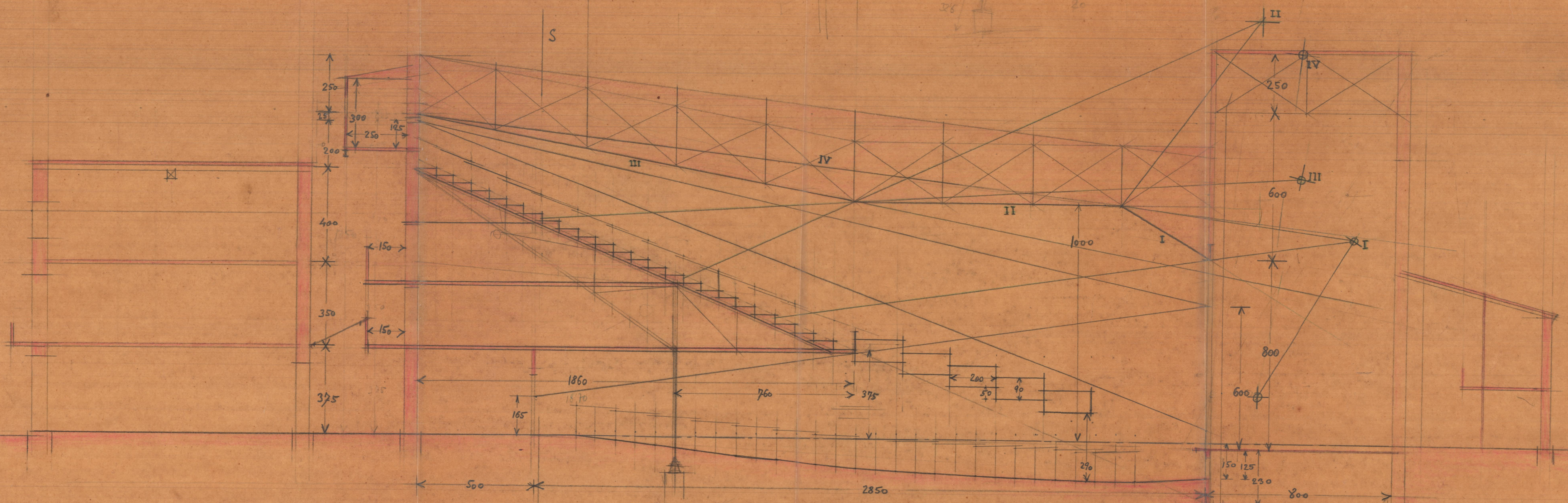
SECCION LONGITUDINAL E. 1:100
