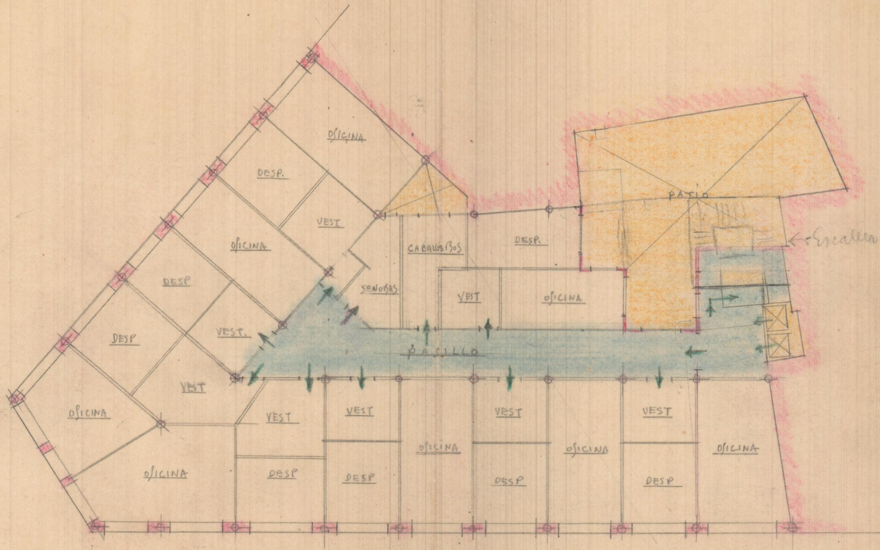
PLANTAS PARA 8 DESPACHOS ESCALERA POR TRANSITO
