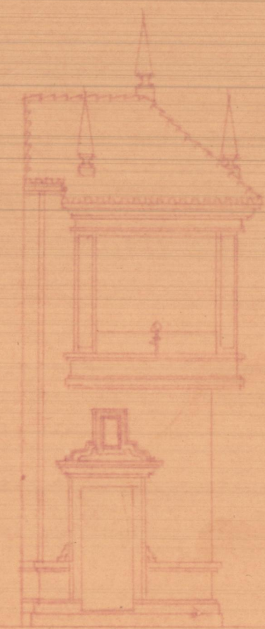
Fachada a Calle 13 Julio
