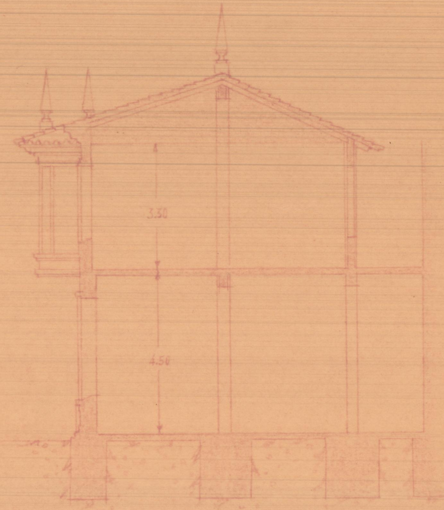
Seccion A-B
