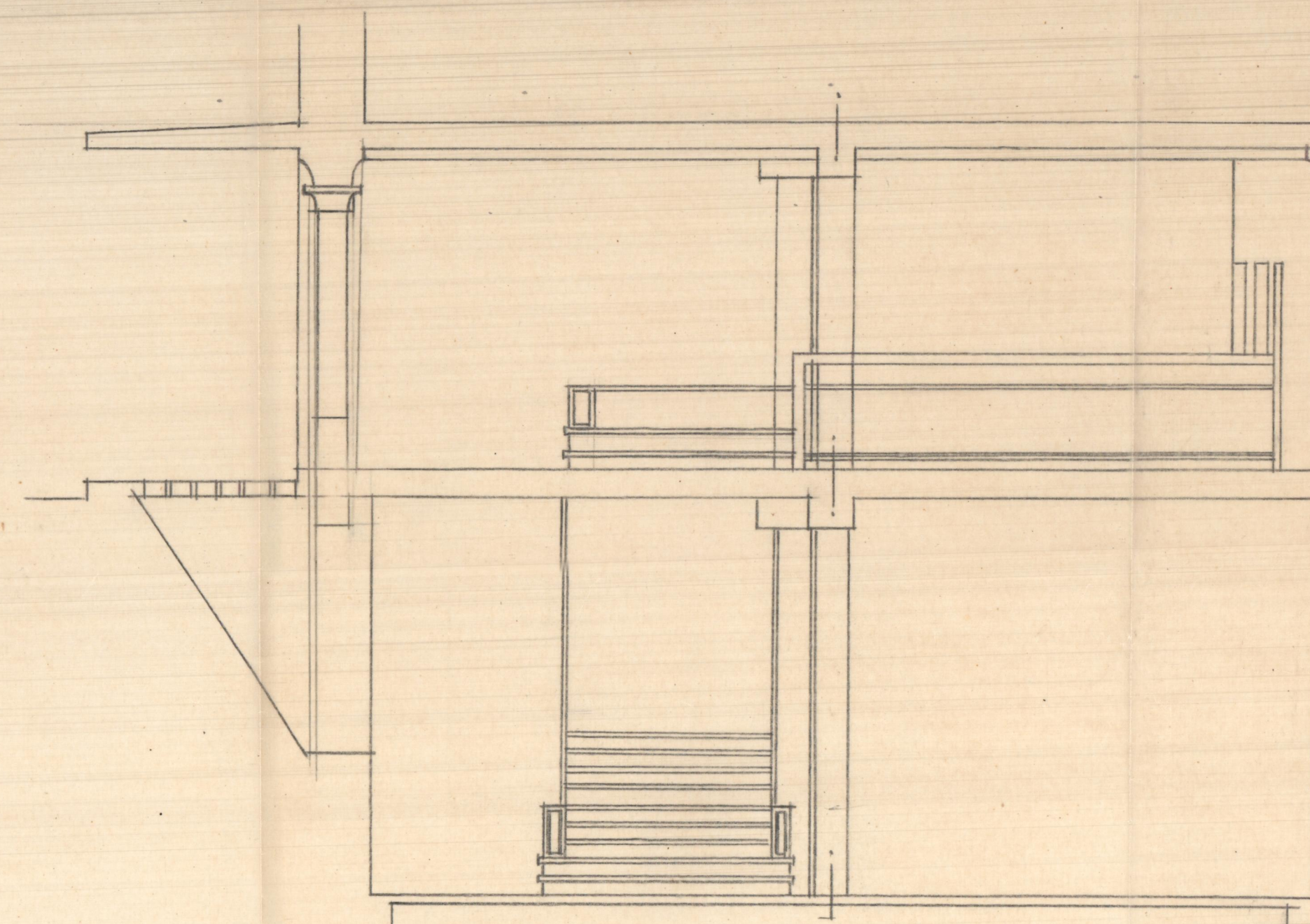
Sección transversal
