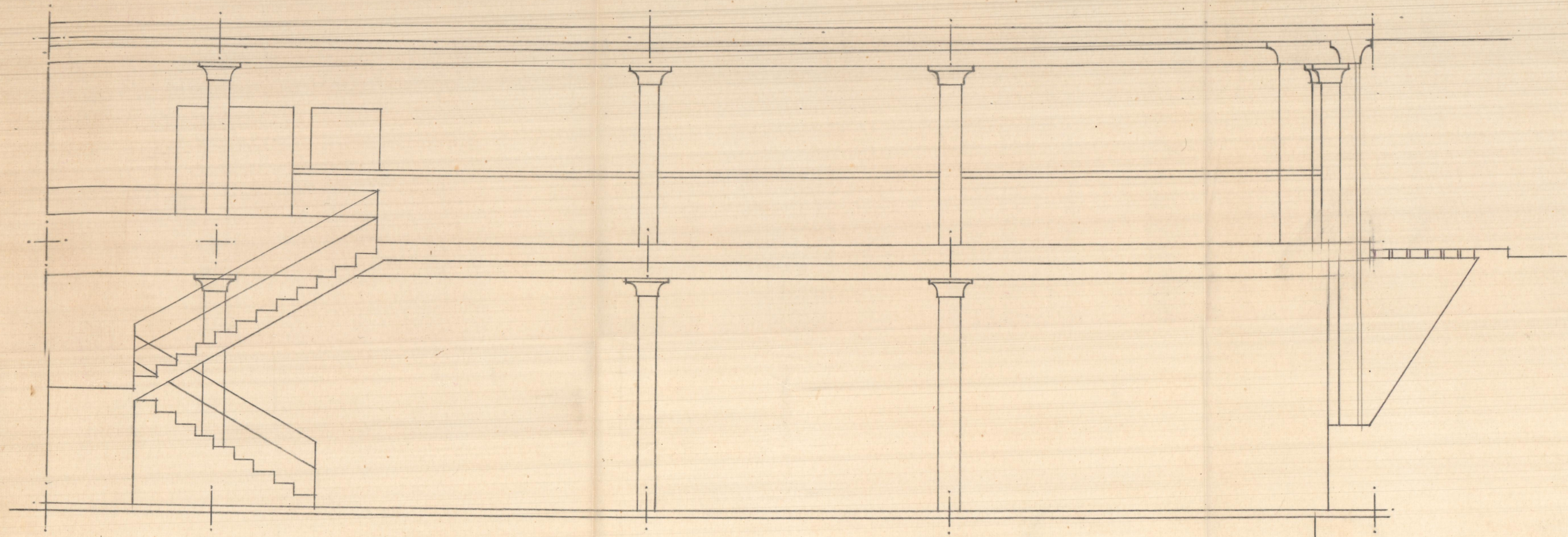
Sección longitudinal
