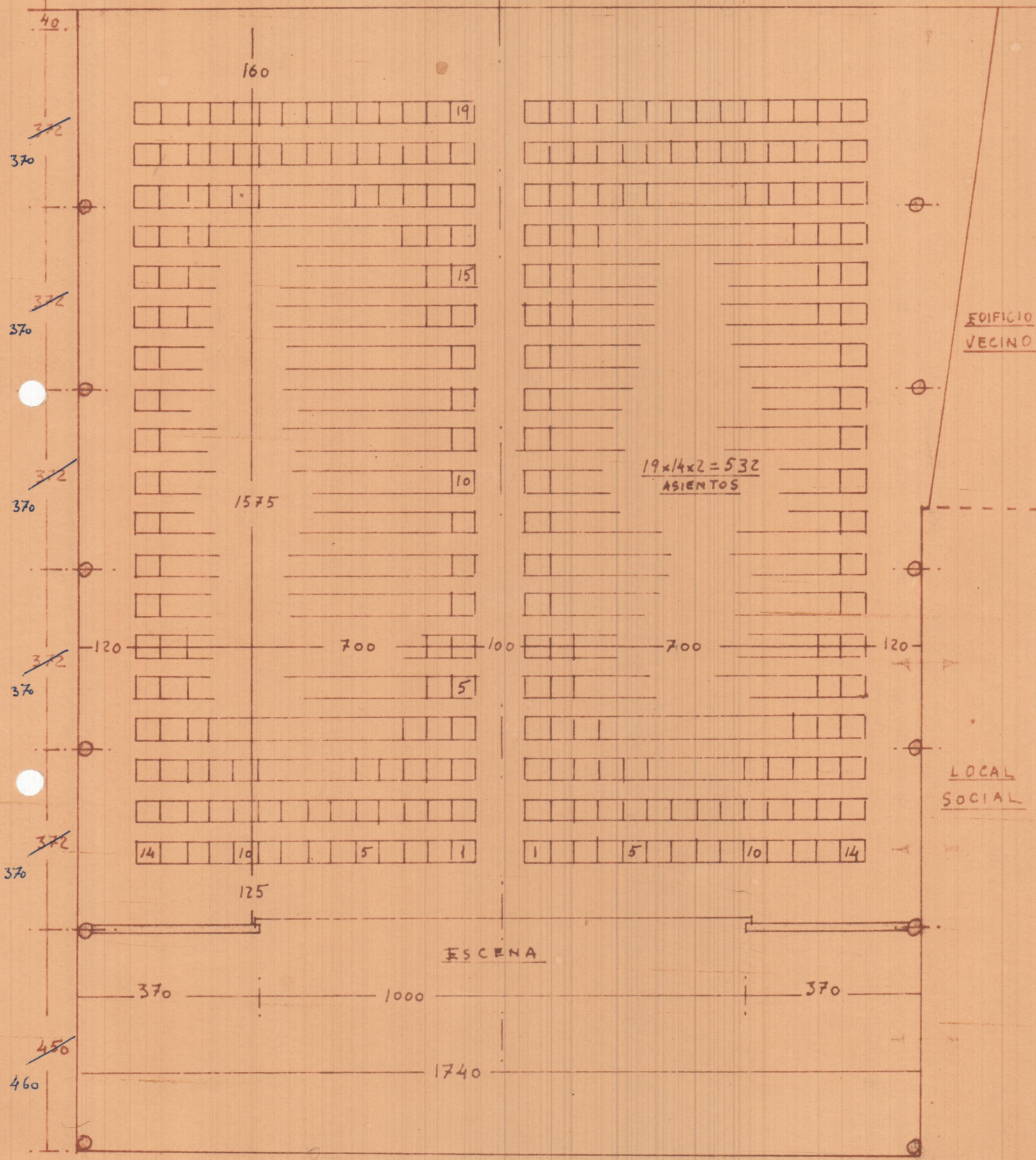
ESCENA INTERIOR - PLANTA - E - 1:100
