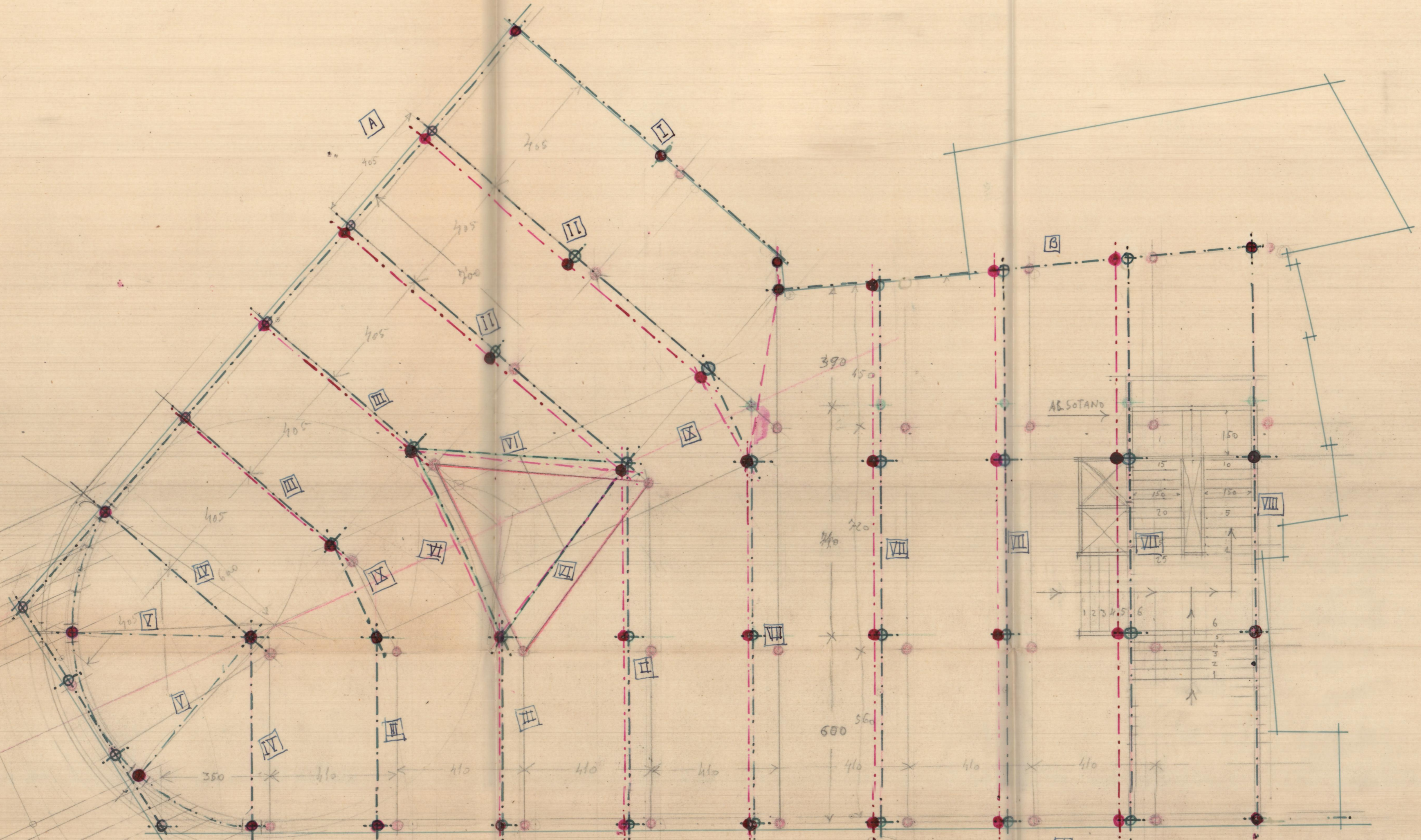
A PLANTA DE ENTRADOS Y CIMENTOS E. J. 100
