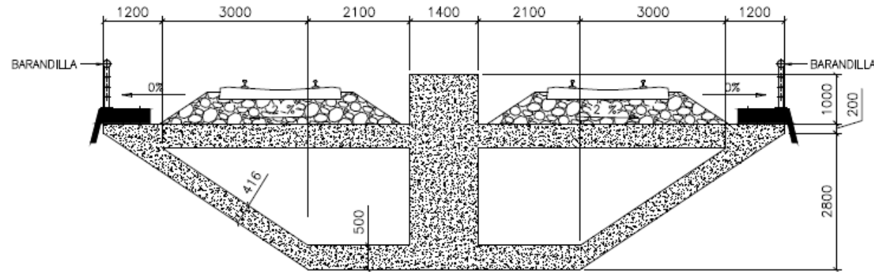
Figura 9.3 Sección transversal en el centro de vano.
