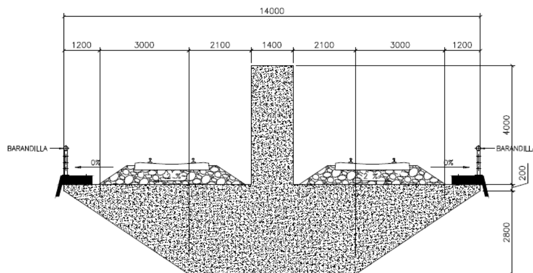
Figura 9.4 Sección transversal sobre las pilas
