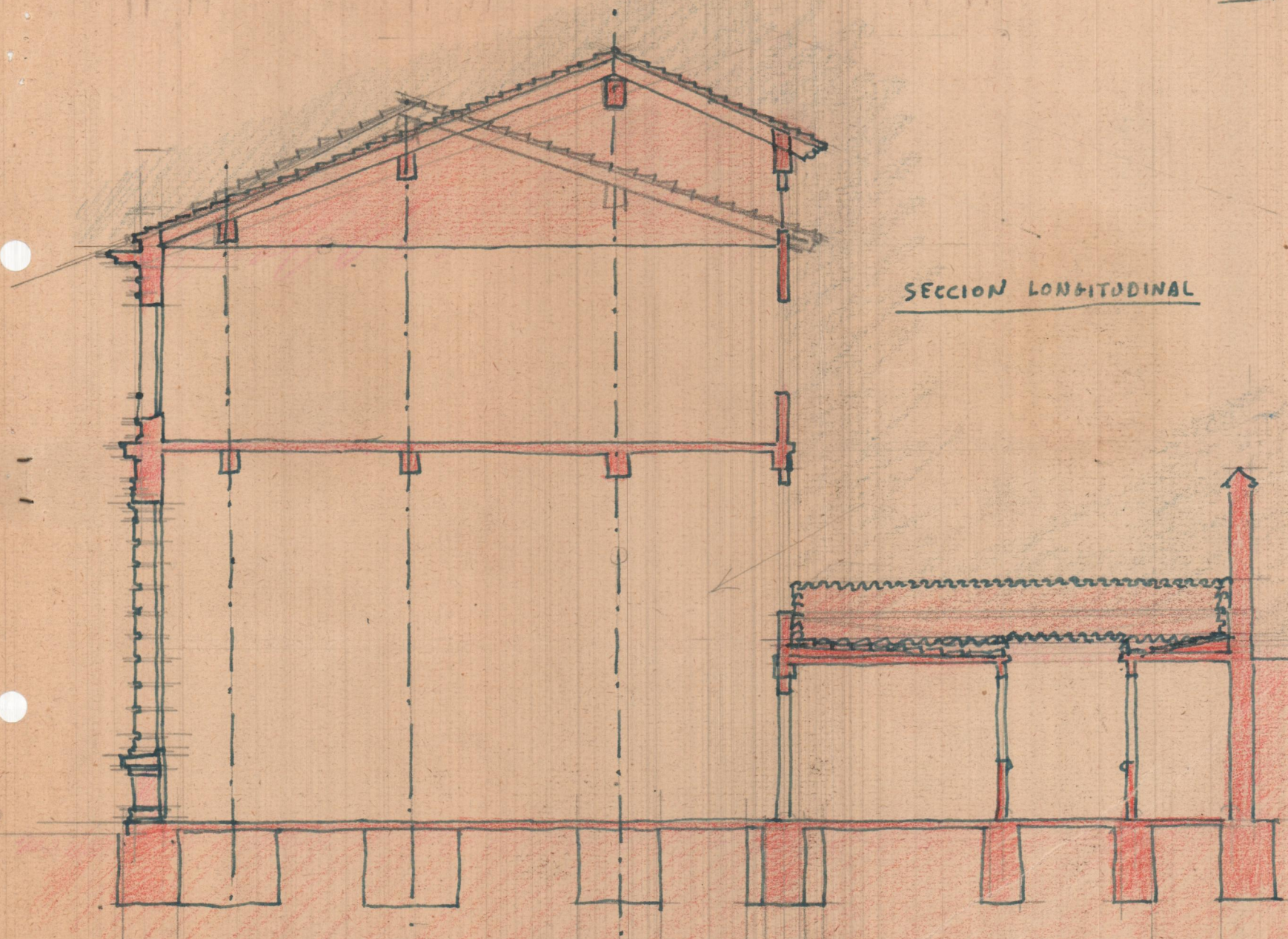
SECCION LONGITUDINAL
