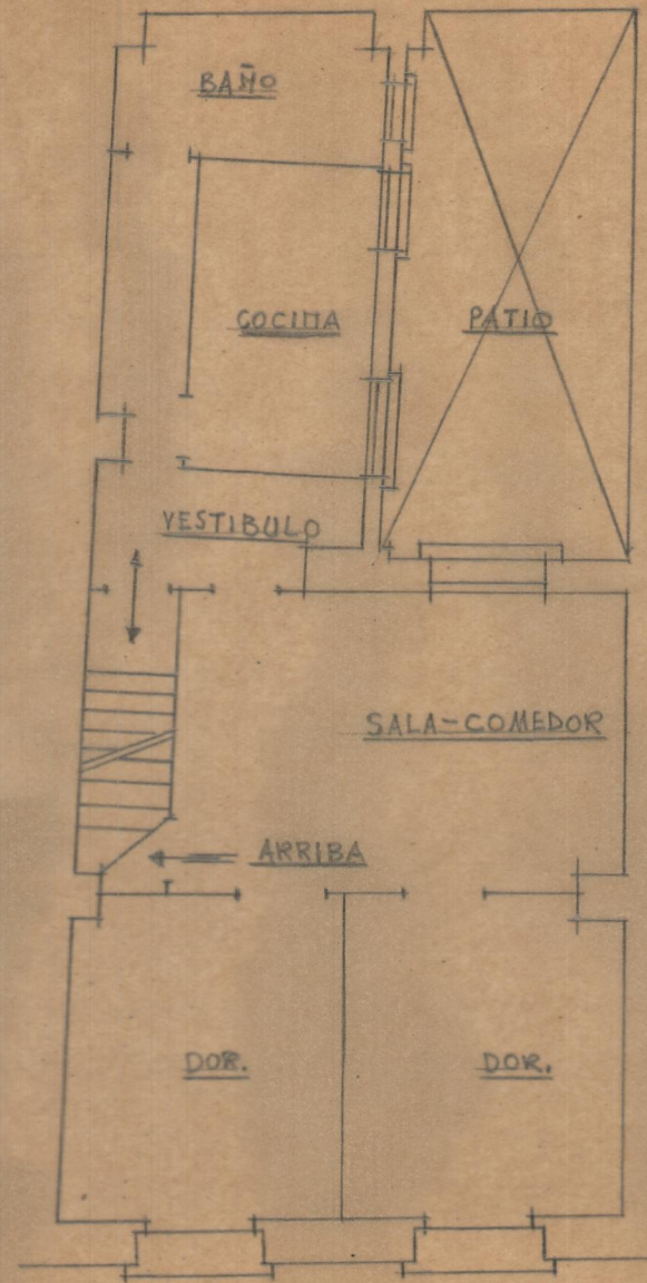
Planta 2ª
